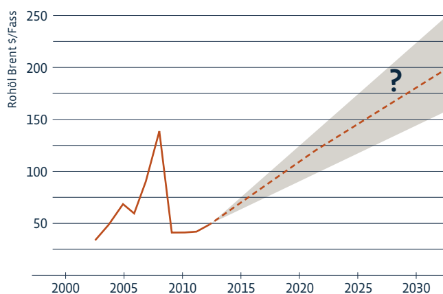
Abbildung 2: Rohölpreis
