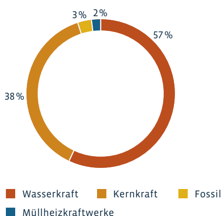
Abbildung 11: Schweizerischer Stromerzeugungsmix 2005
