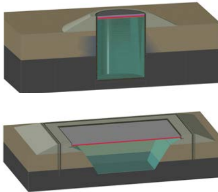
Speichergeometrien, Abb.: Ingenieurbüro ste.p
