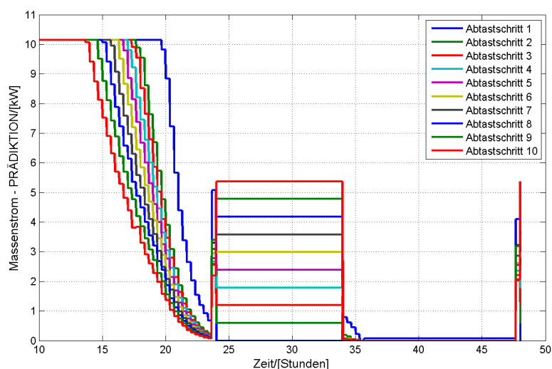
Abbildung 42: Prädizierte Leistungsmodulation - es wird immer der aktuelle Werte auf das System geschaltet und damit das System aktuiert.
