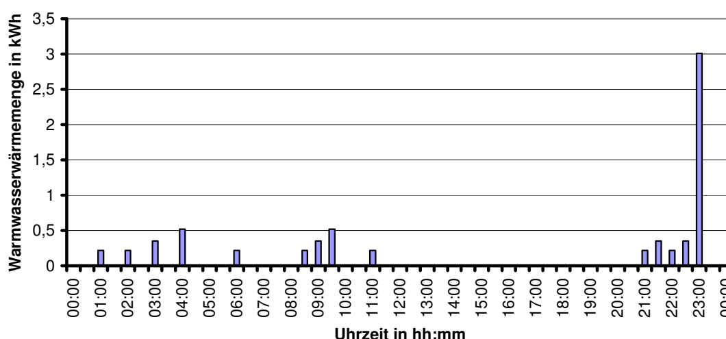
Abbildung 6: Zapfwärmemenge ZP120 nach DIN 4702 Teil 8 mit einer Temperaturspreizung von 36 K
