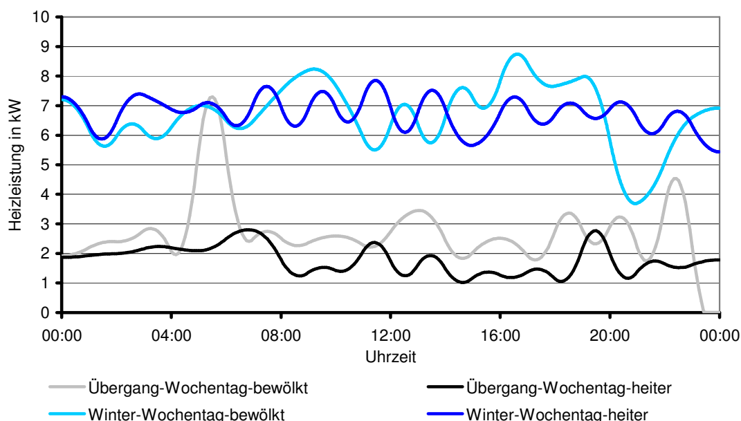
Abbildung 10: Raumwärmebedarfsprofile für bestimmte Typtage nach VDI-Richtlinie 4655 Quelle: VDI-Richtlinie 4655 und eigene Berechnungen
