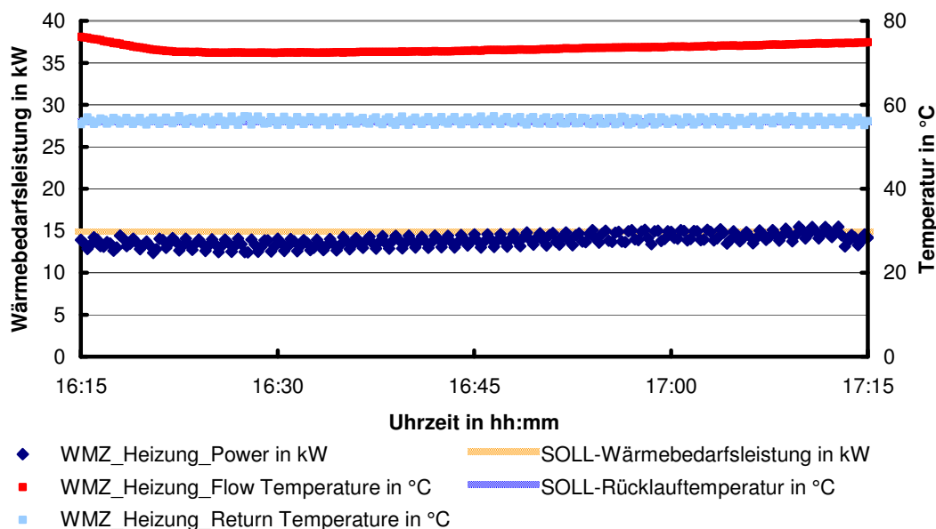
Abbildung 27: Stationärer Betrieb bei 14,9 kW Wärmebedarfsleistung und 56°C Rücklauftemperatur
