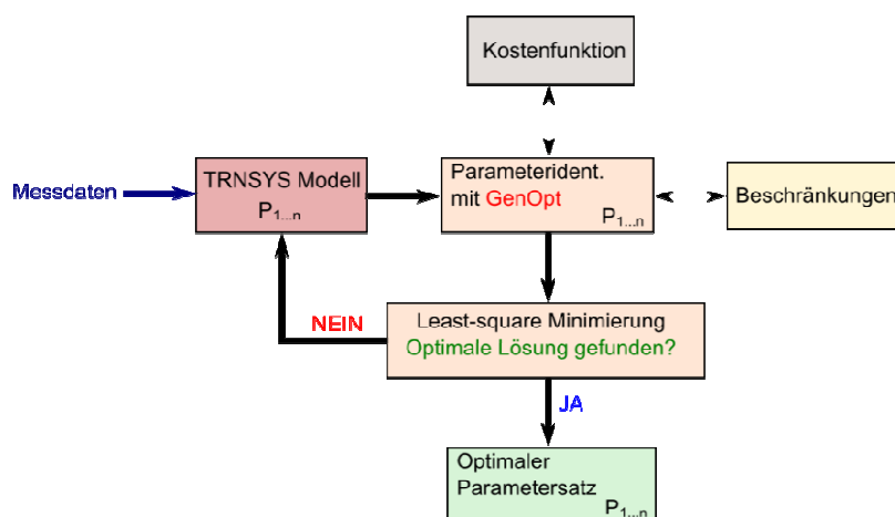
Abbildung 39: Ablaufdiagramm der Parameteroptimierung (Quelle: AIT)
