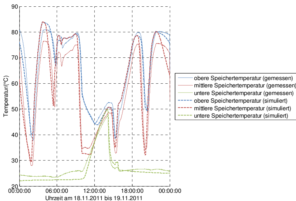
Abbildung 36: Gemessene und simulierte Temperaturverläufe der Anlage Koller
