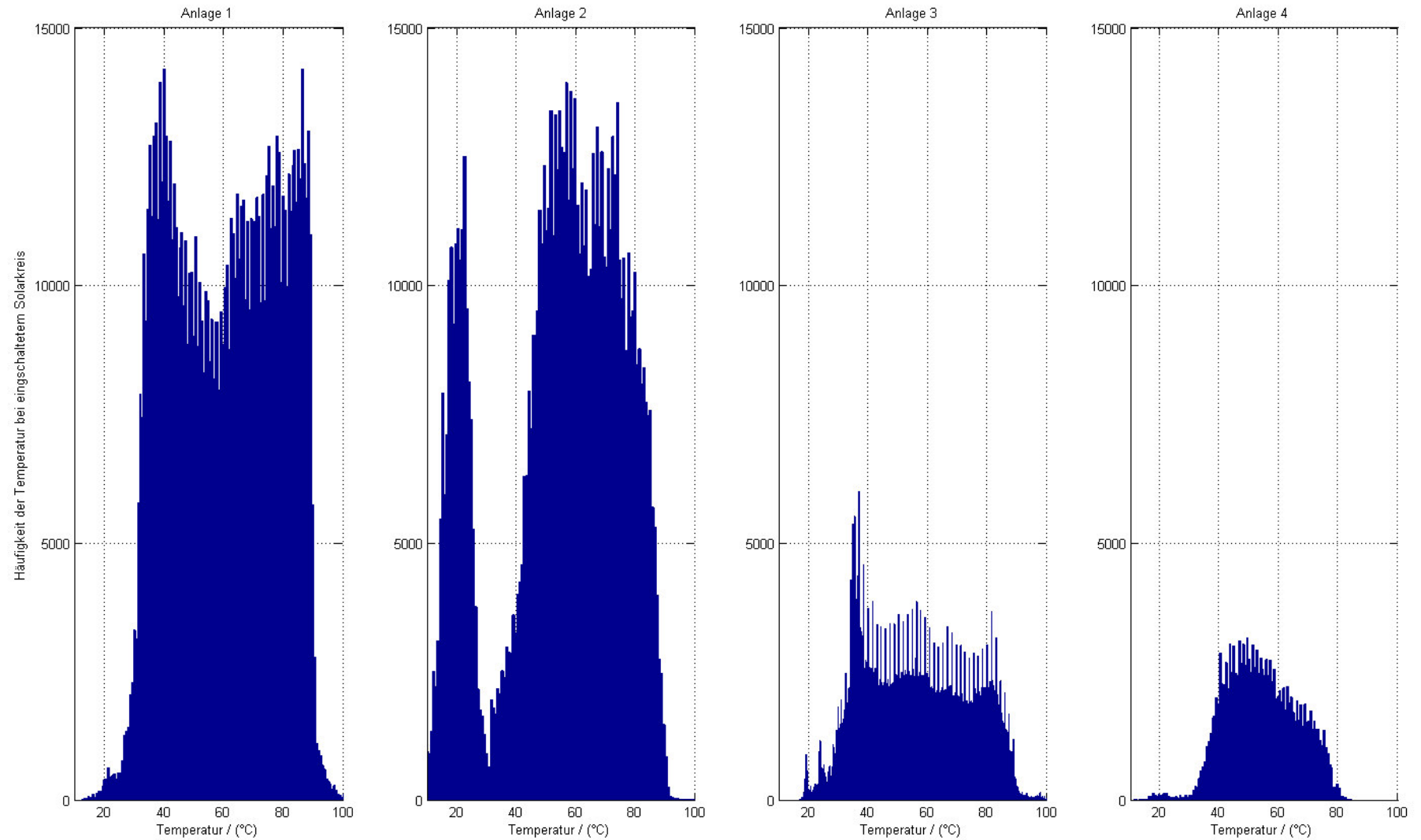
Abbildung 19: Häufigkeit der Liefertemperatur der Solaranlage bei eingeschalteter Solarkreispumpe der Anlagen über den gesamten Messzeitraum
