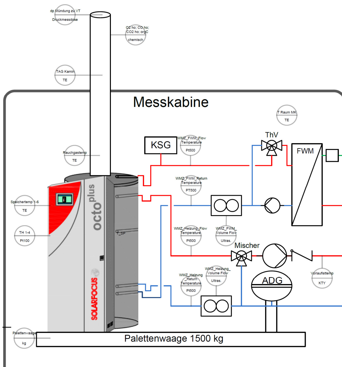
Abbildung 24: Messaufbau für die Labormessungen innerhalb der Messkabine
