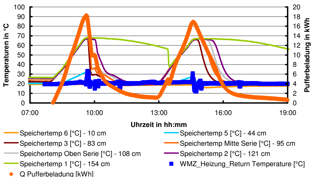
Abbildung 30: Temperaturverläufe und Pufferbeladung bei zweimaliger Be- und Entladung mit Brenner; die Abstände in cm beziehen sich auf die Pufferspeicherunterkante
