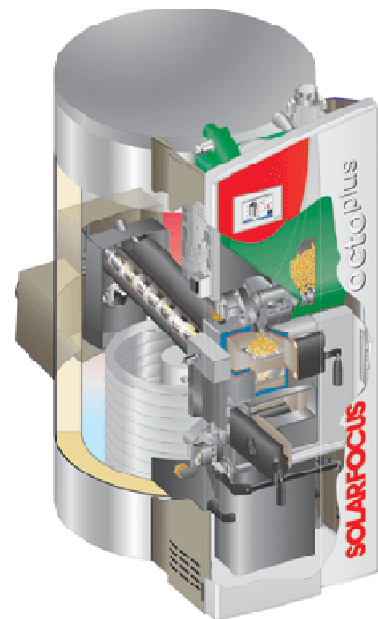
Abbildung 2: Darstellung einer Solarthermie-Biomasse Kompakteinheit 7
