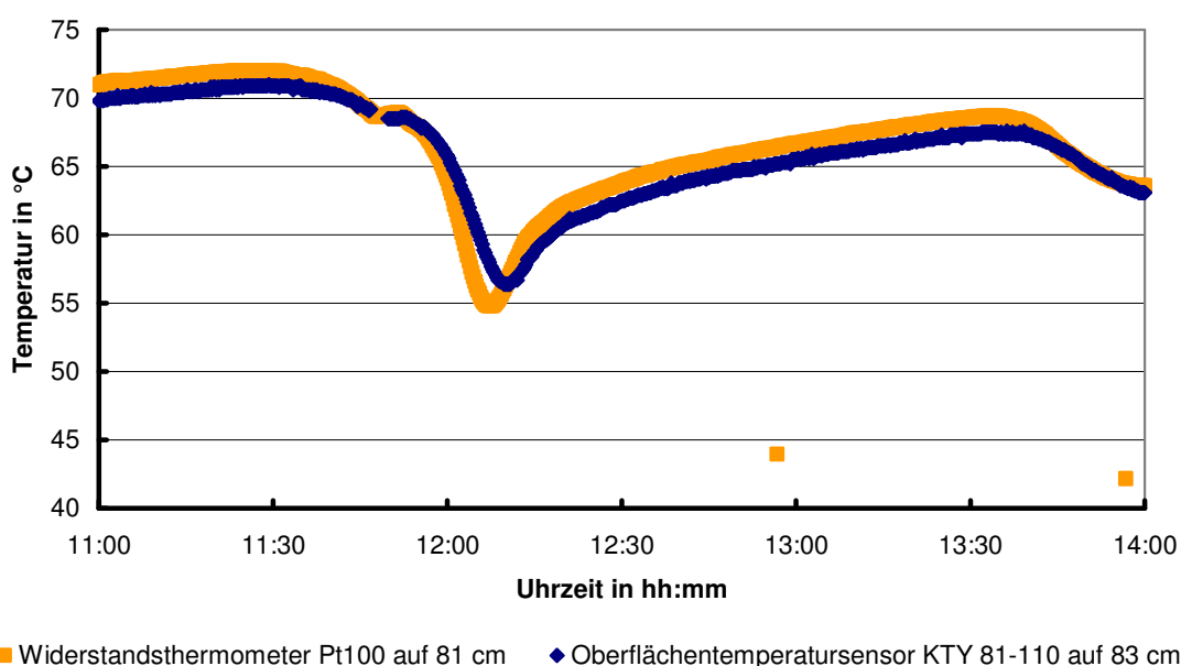
Abbildung 32: Vergleich der Temperaturmesssensoren Pt100 in der Tauchhülse und des Oberflächentempertursensors KTY 81-110.
