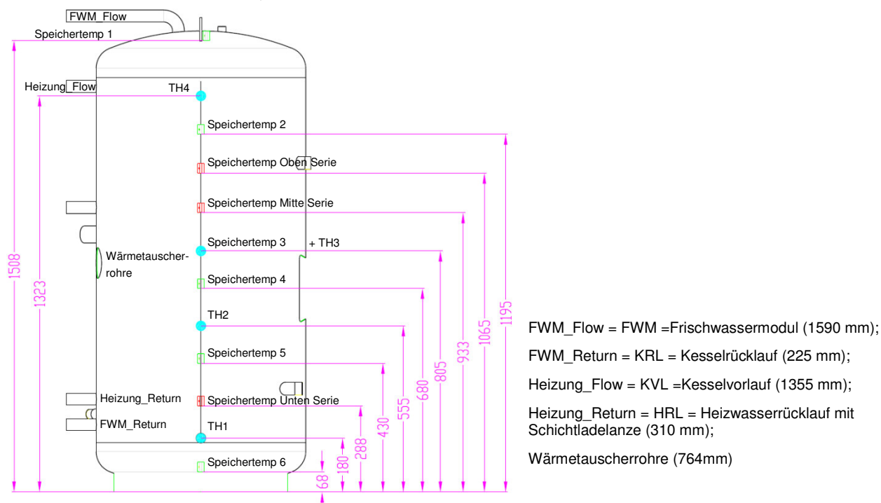
Abbildung 25: Geometrie des Pufferspeichers und Dokumentation der Temperaturfühler; Angaben in mm
