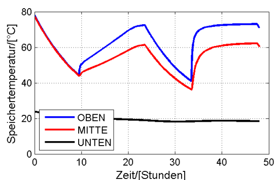
Abbildung 41: Speichertemperaturen unter Einsatz modellprädiktiver Regelung.
