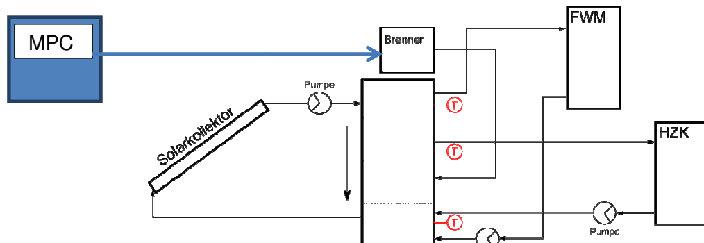
Abbildung 38: KOMBINE System Konfiguration: drei entkoppelte Regelkreise (Solar, Frischwasser (FWM) und Heizung (HZK)) - MPC dient überlagert als Energiemanagement für die unterlagerten Regelkreise und greift dabei in die Brennermodulation ein um diese optimal zu gestalten.
