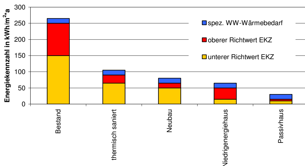
Abbildung 12: Energiekennzahl und spez. Warmwasserwärmebedarf unterschiedlicher Gebäudetypen Quelle: eigene Berechnungen
