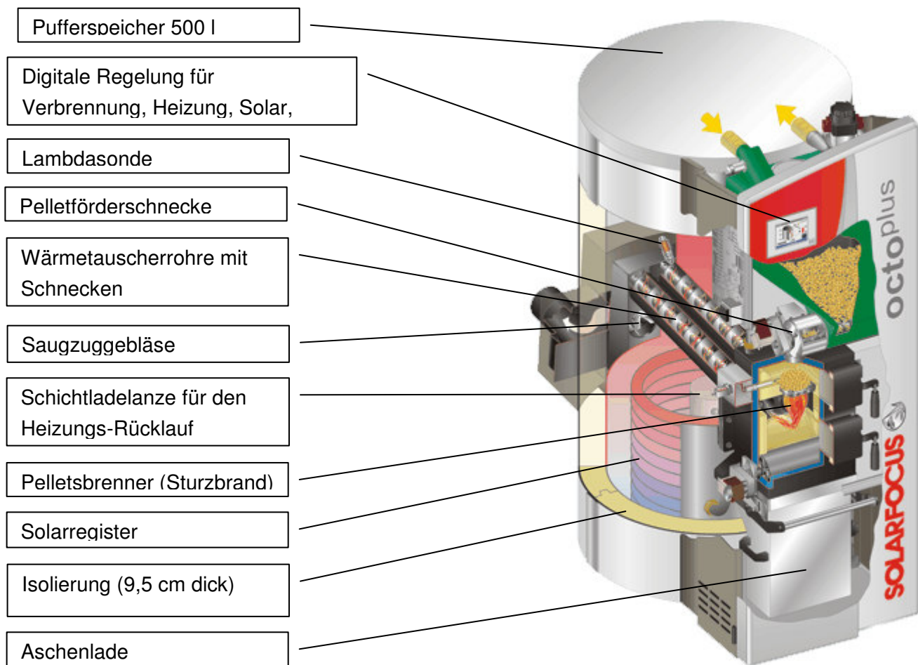
Abbildung 23: Schnittbild der Versuchsanlage octo plus von solarfocus mit Bezeichnung von Einzelteilen
