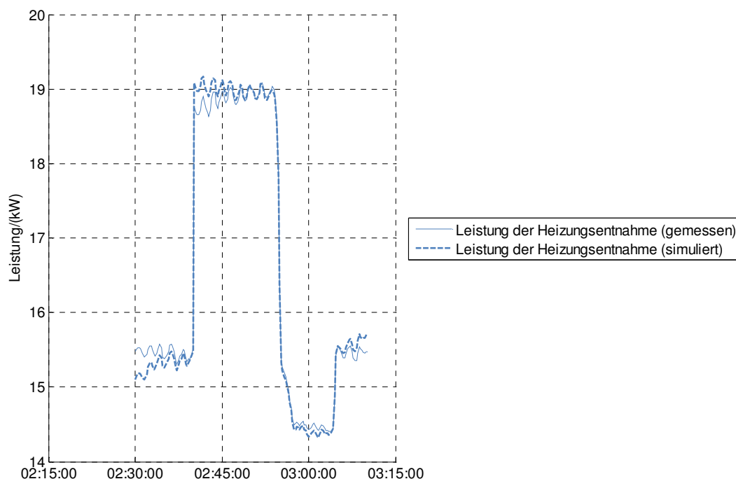
Abbildung 35: Gemessene und simulierte Leistungen beim Laborversuch mit 75% Leistung und 30°C Rücklauftemperatur
