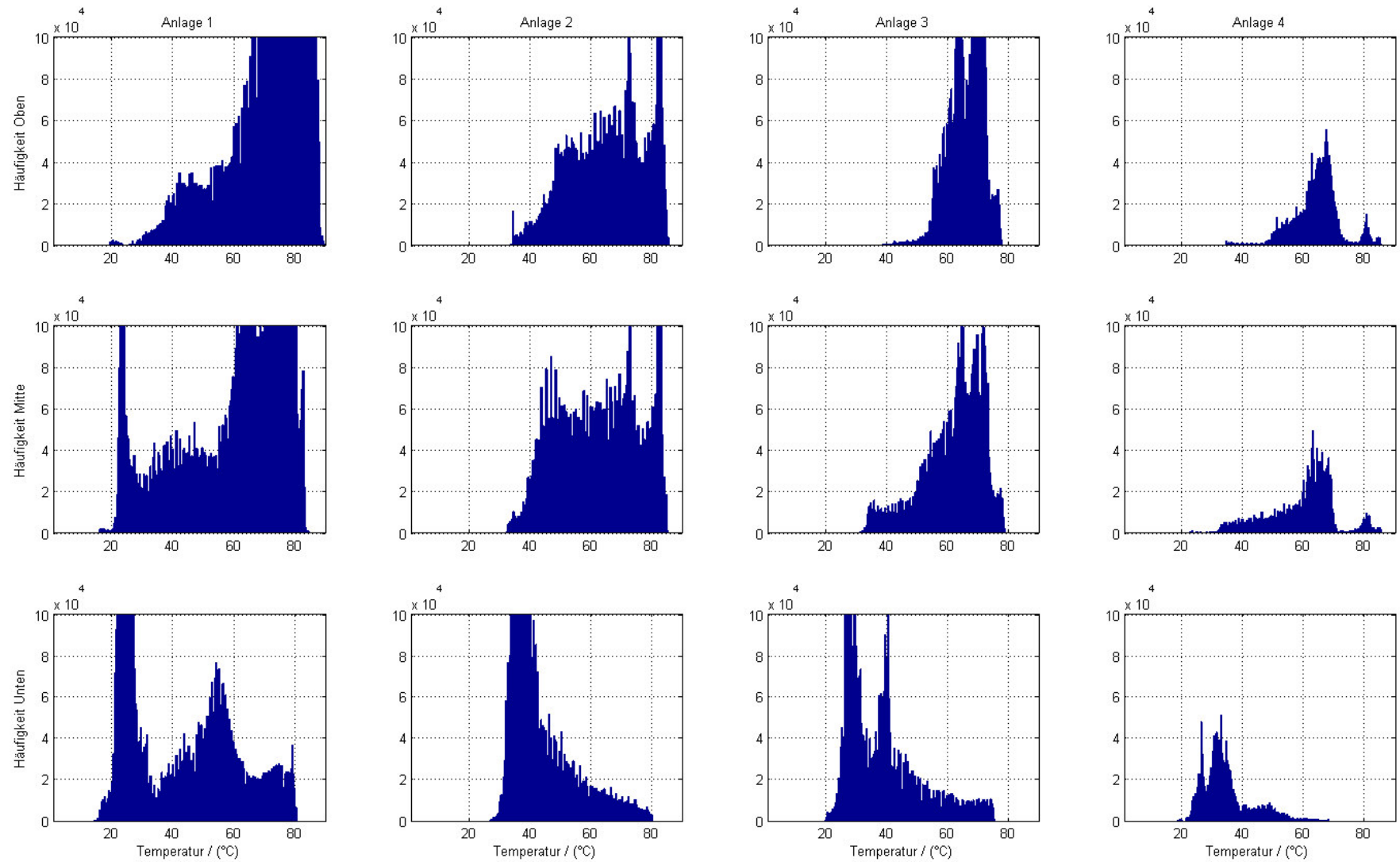
Abbildung 18: Häufigkeit der Speichertemperaturen der Anlagen über den gesamten Messzeitraum
