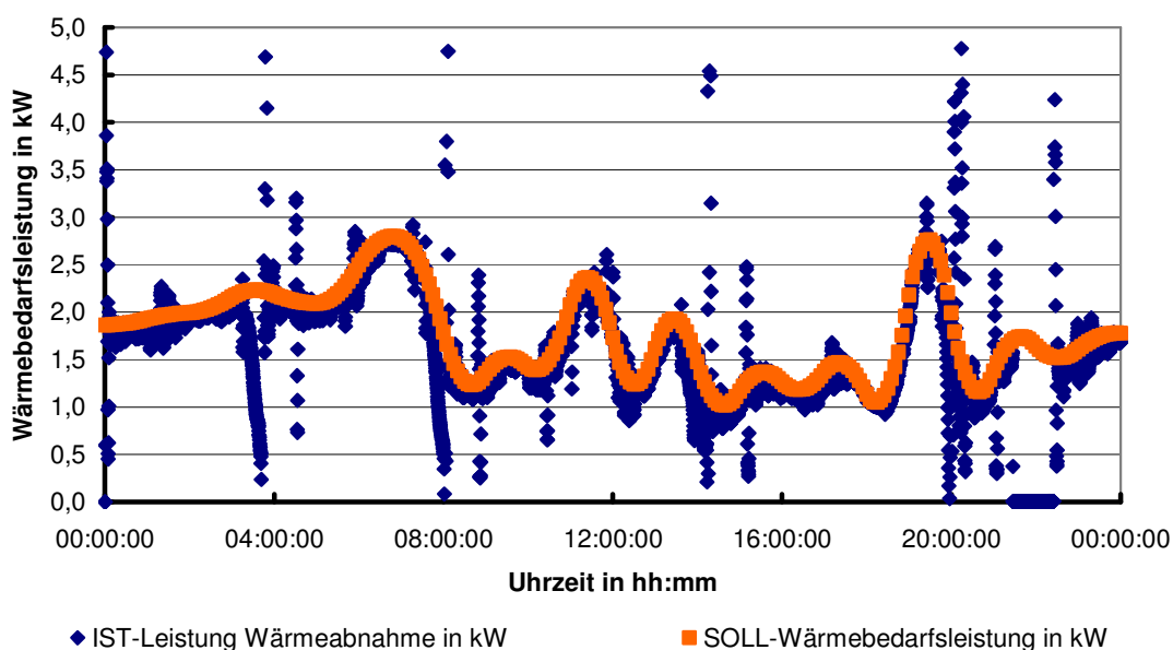
Abbildung 29: Vergleich der SOLL-Wärmebedarfsleistung mit der IST-Leistung Wärmeabnahme des Lastprofils ÜWH
