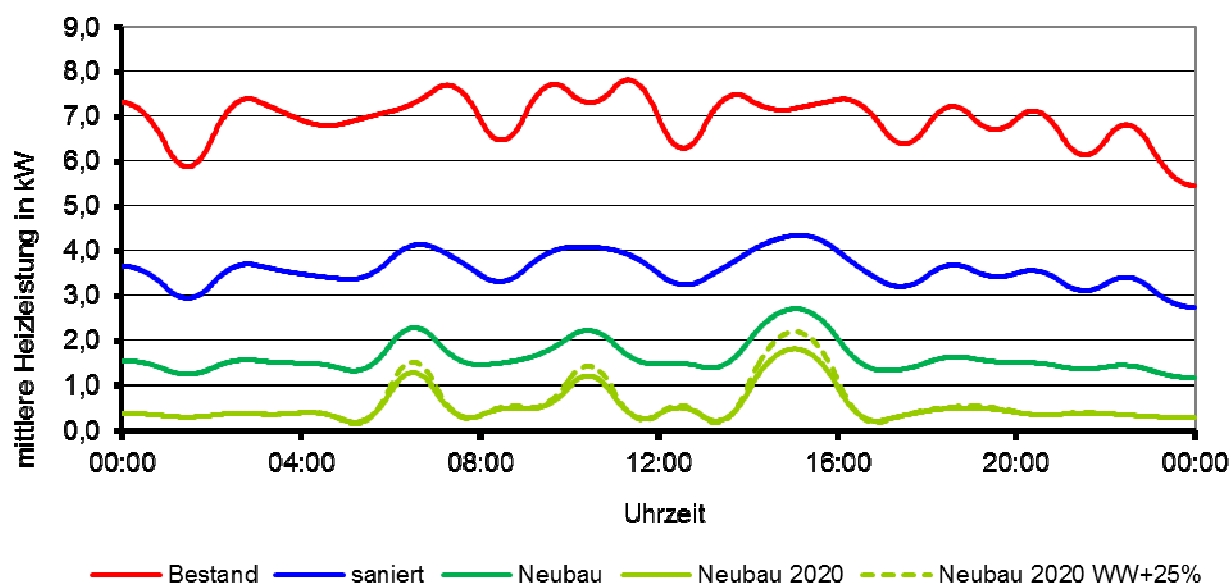
Abbildung 11: Wärmebereitstellungsprofile in Abhängigkeit des Gebäudestandards für den Typtag: Winter-Wochentag-heiter
