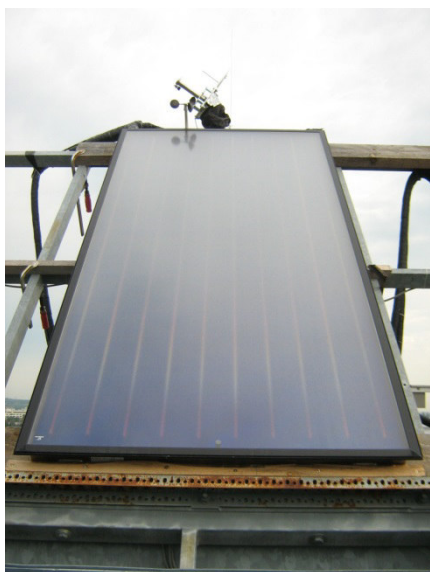
Abbildung 21: Aufbau Solarkollektor auf dem Prüfstand (Quelle: AIT)
