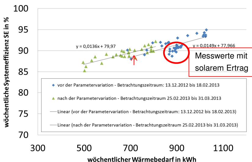
Abbildung 43: Ergebnis der Parametervariation bei Berücksichtigung des Wärmebedarfes
