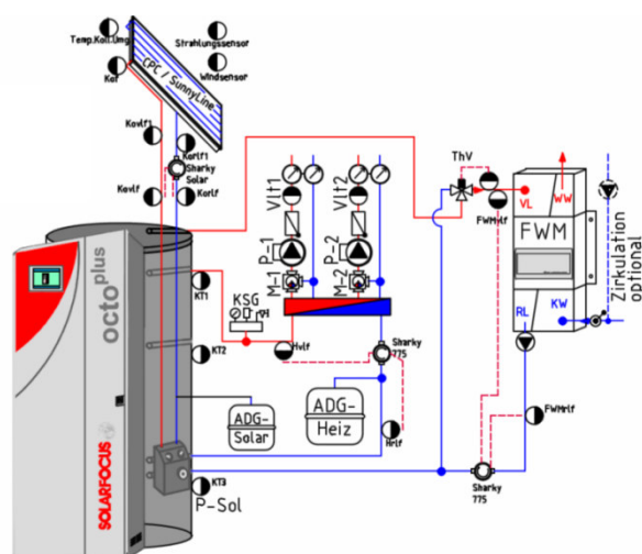
Abbildung 13: Monitoring – Hydraulisches und elektrisches Schema für die drei Objekte am Feld (Quelle: Solarfocus)
