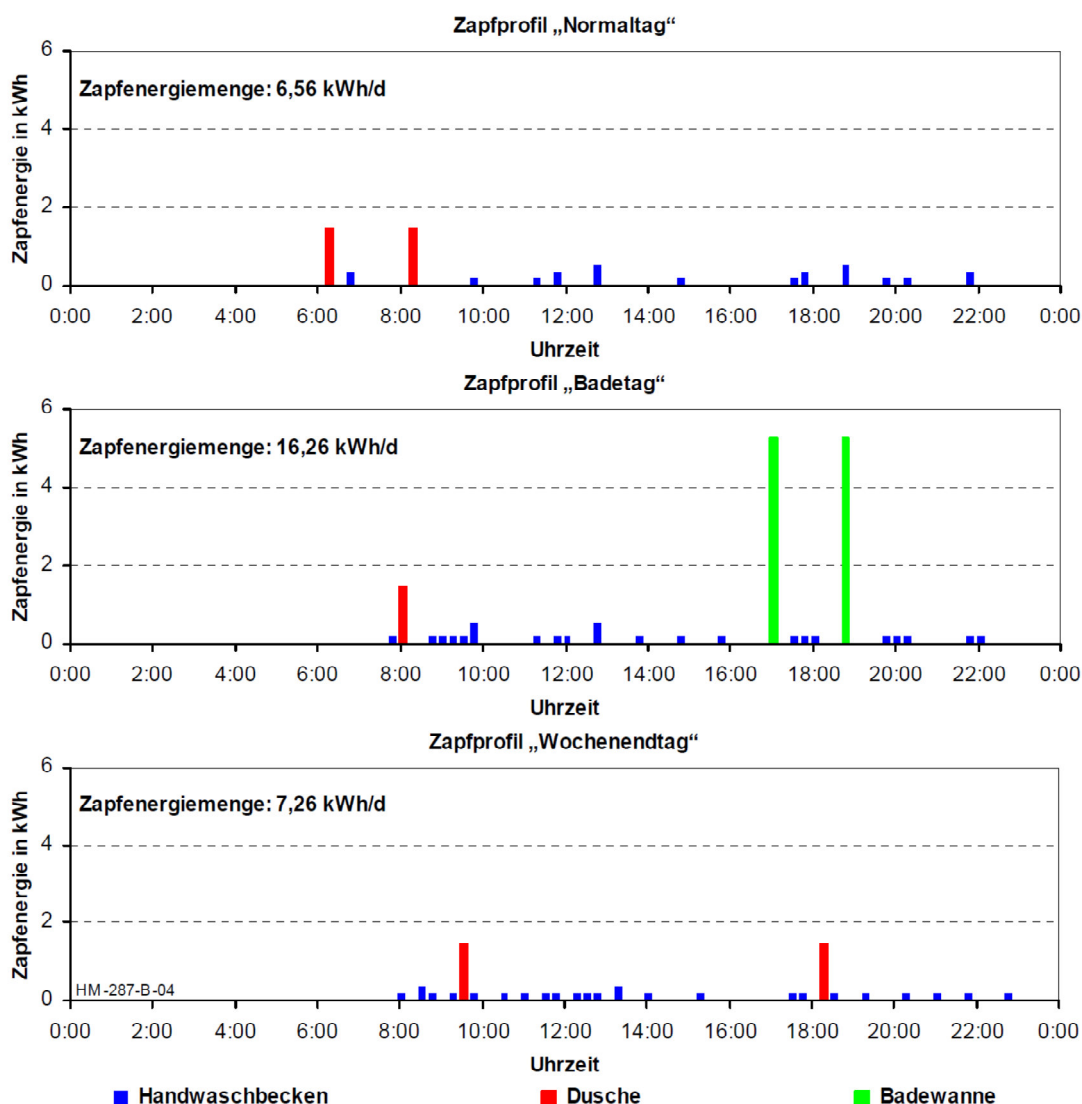
Abbildung 8: Warmwasserwärmebedarfsprofile für Normaltag, Badetag und Wochenende für einen Drei- bis Vierpersonenhaushalt in Abhängigkeit vom Zapfstellentyp
