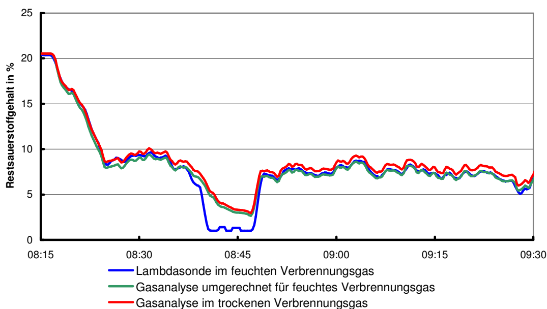
Abbildung 31: Vergleich des Restsauerstoffgehalts gemessen mittels Lambdasonde und Gasanalyse
