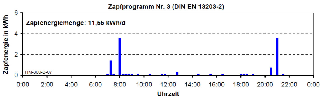
Abbildung 7: Zapfwärmemenge nach Zapfprogramm Nr.3 für Küche, Dusche und Baden
