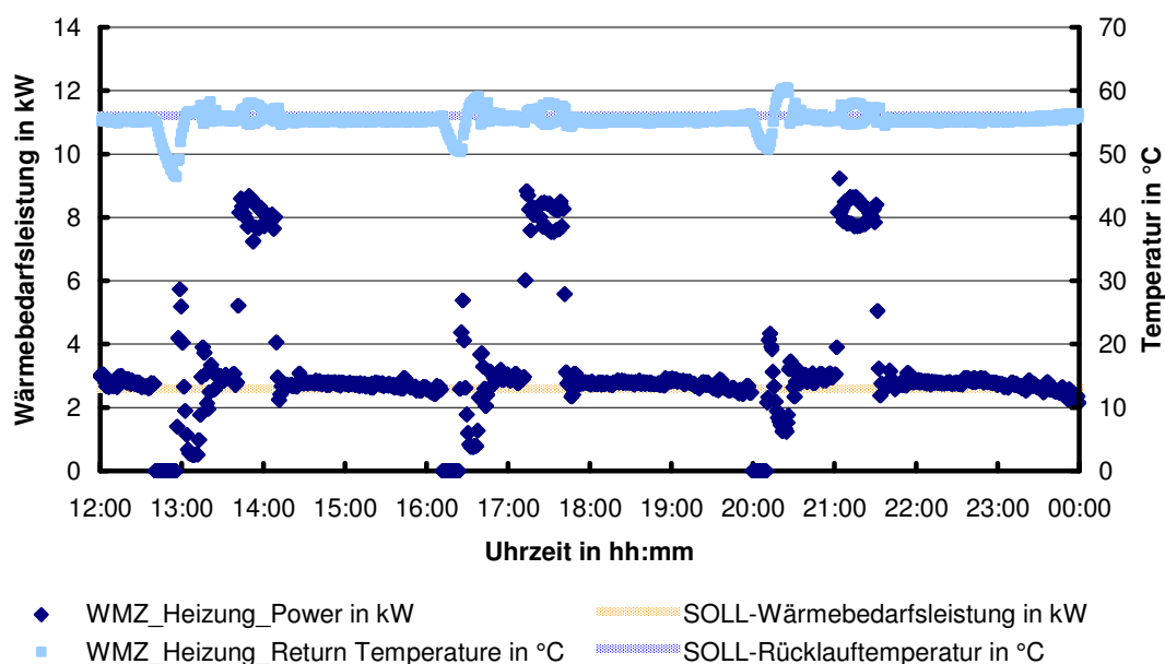
Abbildung 28: Intermittierender Betrieb bei 2,6 kW Wärmebedarfsleistung und 56 °C Rücklauftemperatur
