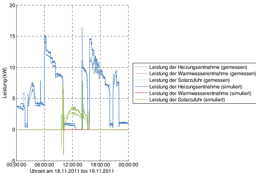
Abbildung 37: Gemessene und simulierte Leistungen der Anlage Koller
