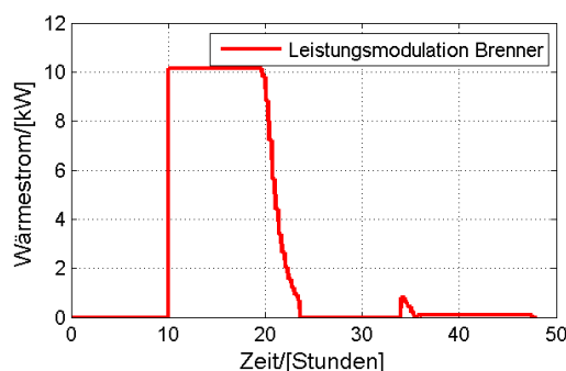
Abbildung 40: Leistungsmodulation für den Brenner - mit modellbasierter, prädiktiver Regelung.
