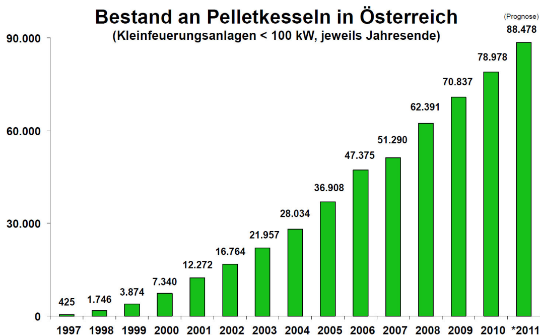
Abbildung 2: Bestand an Pelletskesseln in Österreich bis 100 kW von 1997 bis 2011
