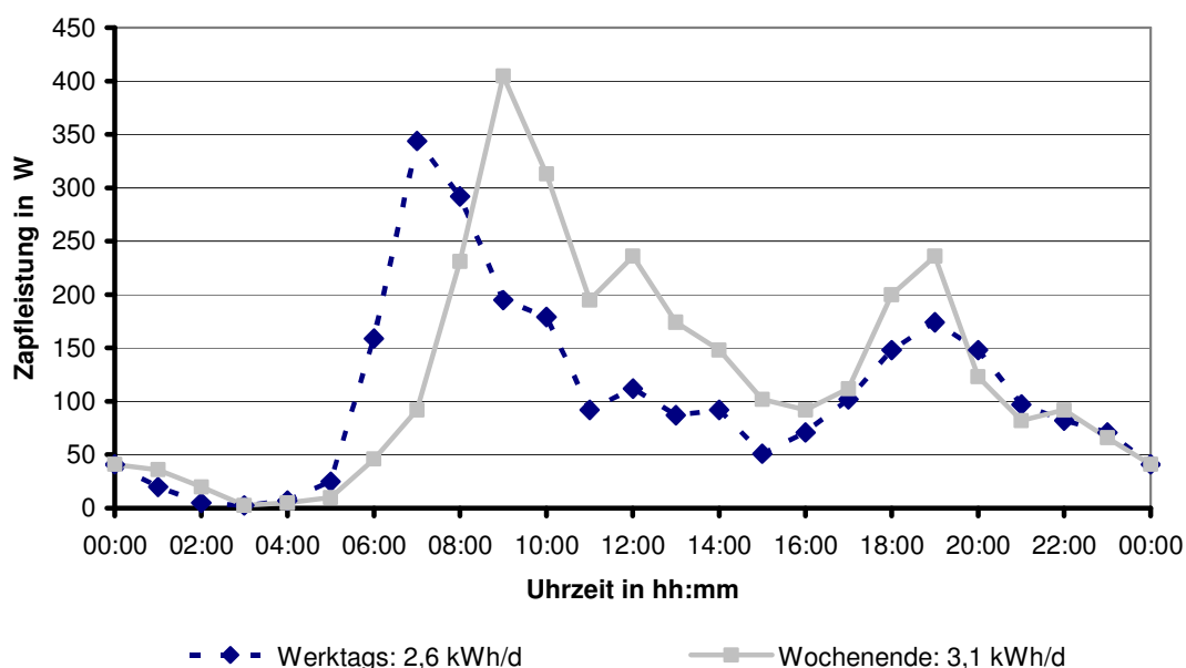
Abbildung 4: Mittlerer Tagesprofil für einen Jahreswarmwasserbedarf von 1 MWh pro Person Quelle: MUEHLBACHER, CARTER 2002
