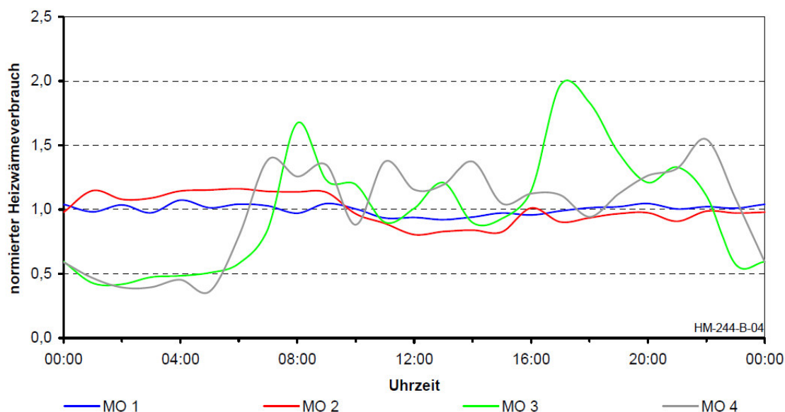
Abbildung 9: normierter Heizwärmebedarf von untersuchten Ein- und Zweifamilienhäuser sowie Reihenhäuser bezogen auf den Stundenmittelwert des Tagesverbrauchs an Werktagen Quelle: [MUEHLBACHER 2008]
