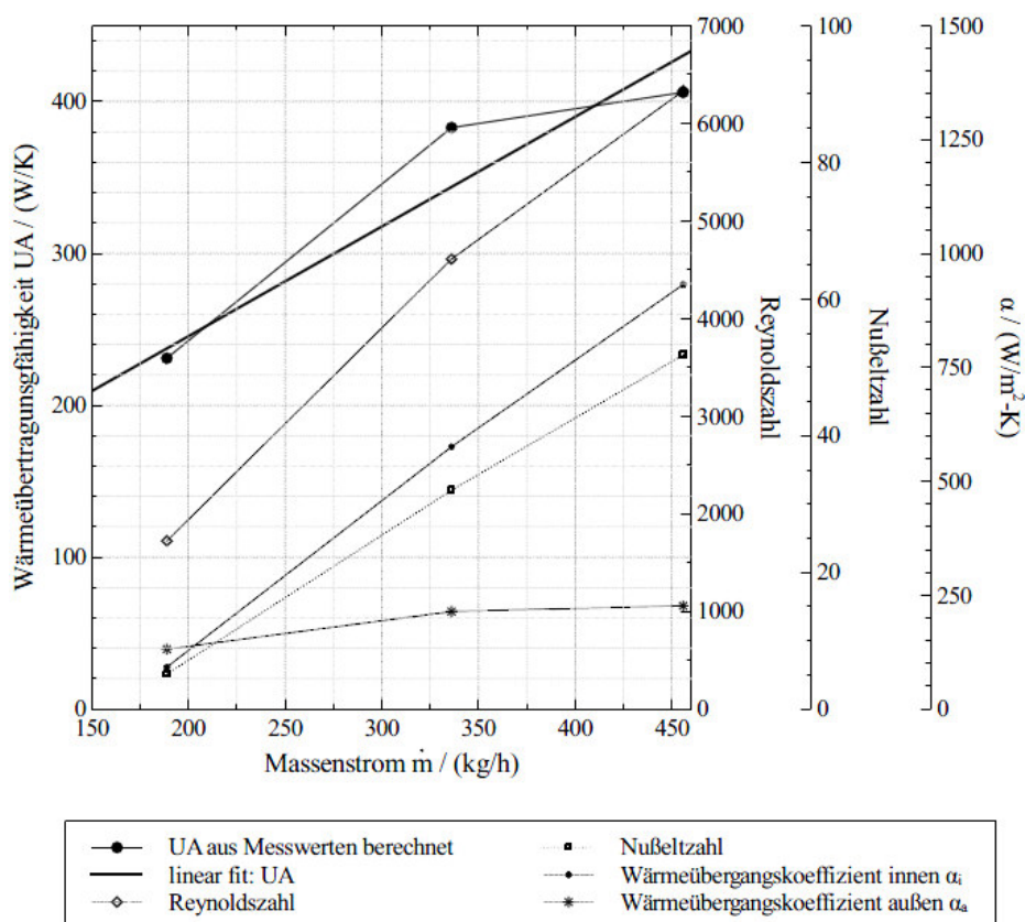
Abbildung 22: Ausgewertete Wärmeübertragungsfähigkeit aus den Messreihen für den Solarwärmeübertrager im Zuge der erweiterten Labormessung an der vierten Anlage
