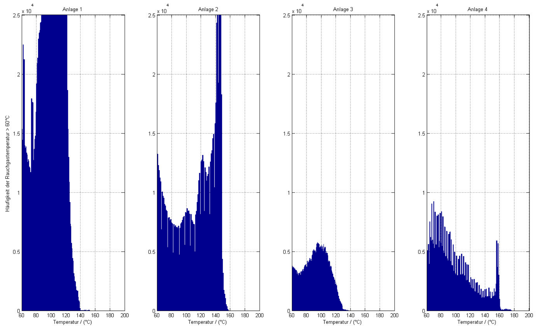
Abbildung 20: Häufigkeit der Rauchgastemperaturen größer 60°C am Austritt aus dem Rauchgaswärmeübertrager im Speicher der Anlagen über den gesamten Messzeitraum
