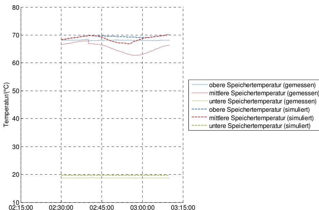
Abbildung 34: Gemessene und simulierte Temperaturverläufe beim Laborversuch mit 75% Leistung und 30°C Rücklauftemperatur
