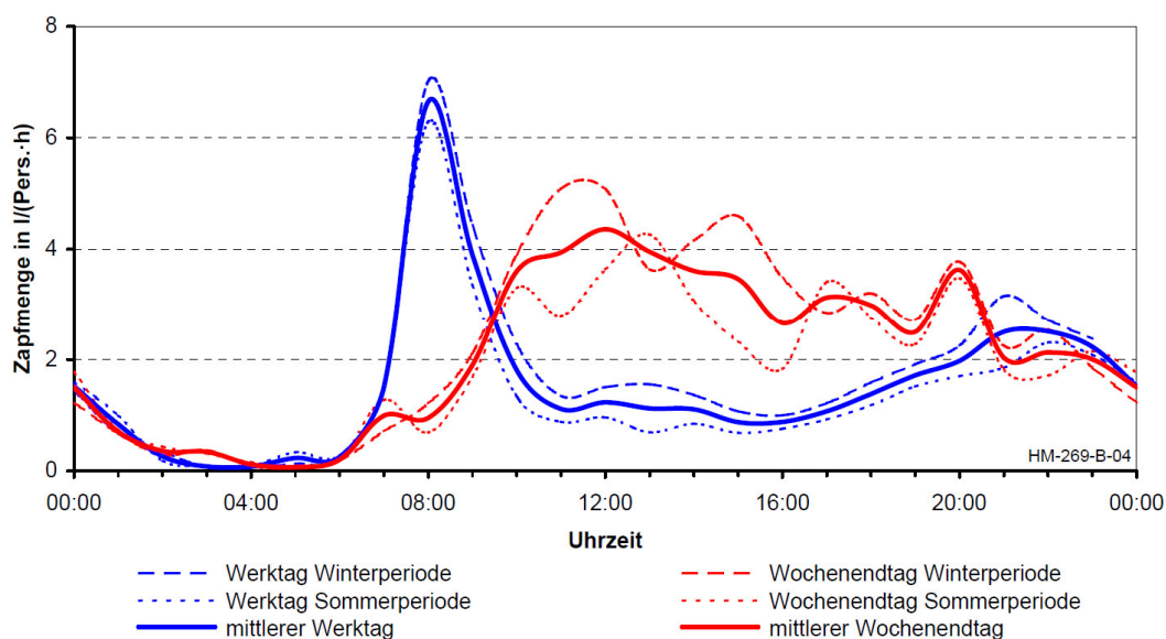
Abbildung 5: Mittlerer Tagesgang der Zapfmenge für die Winter- und Sommerperiode, unterteilt in Werk- und Wochenendtag für ein Mehrfamilienhaus
