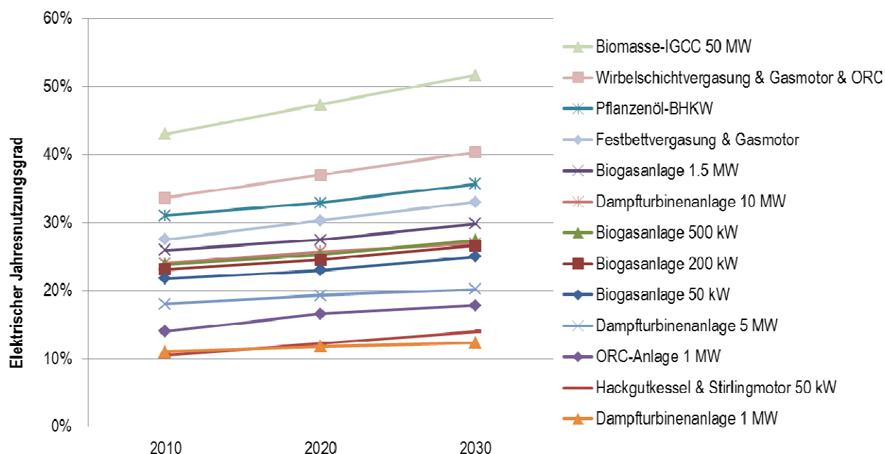
Abbildung 17 Elektrische Wirkungsgrade der Bioenergie-KWK-Technologien Quellen: s. Tabelle 3, Steigerungsraten basieren auf Öko-Institut (2010)
