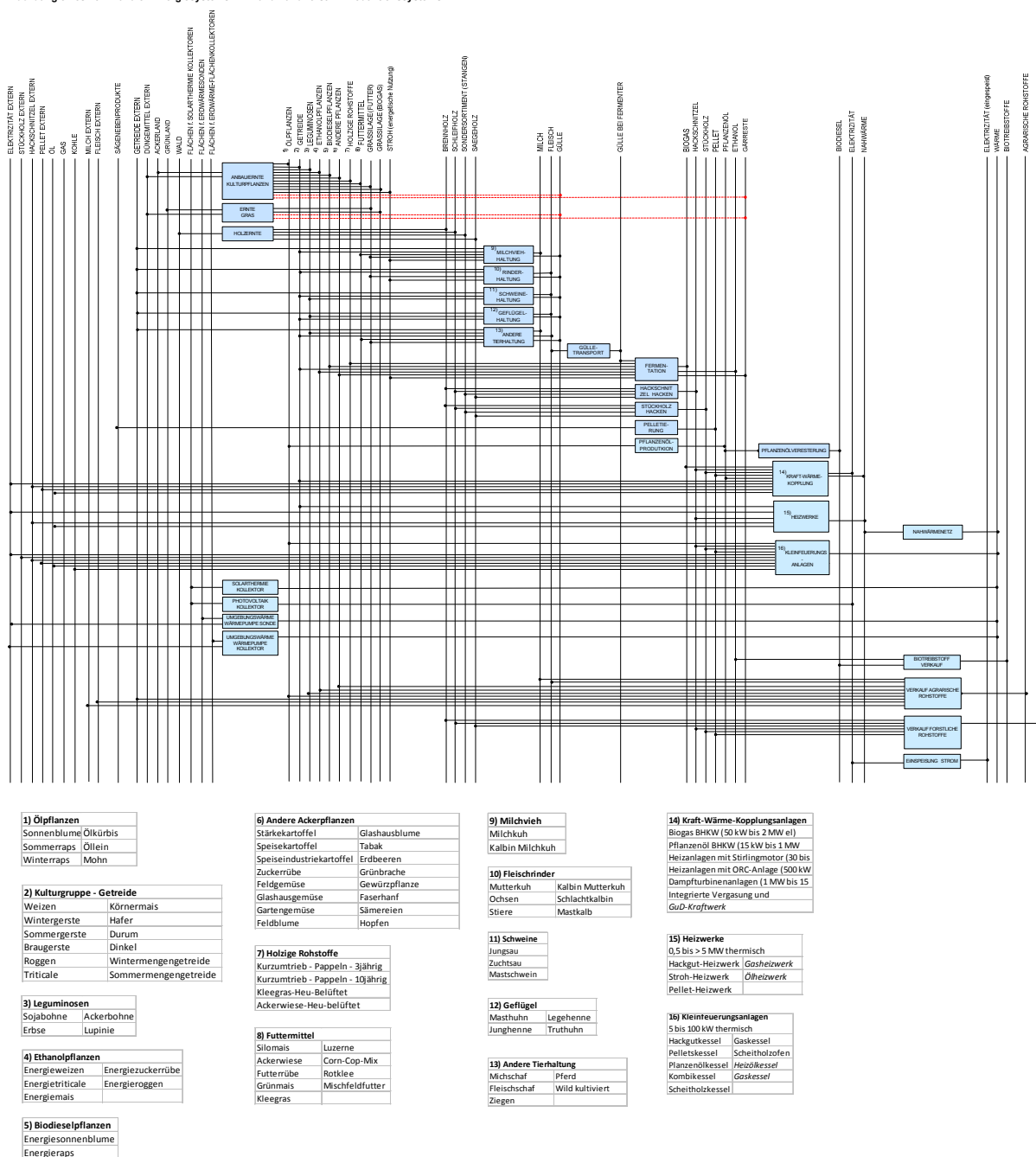
Abbildung 3 Referenzenergiesystem
