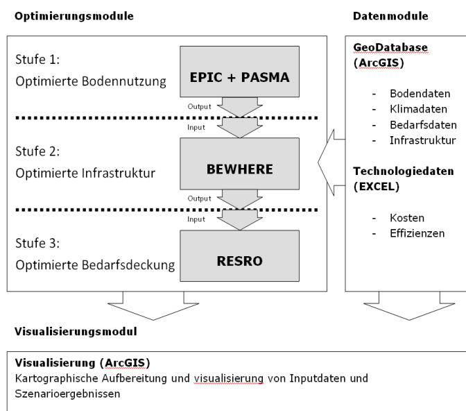
Abbildung 7 Optimierungsmodellverbund
