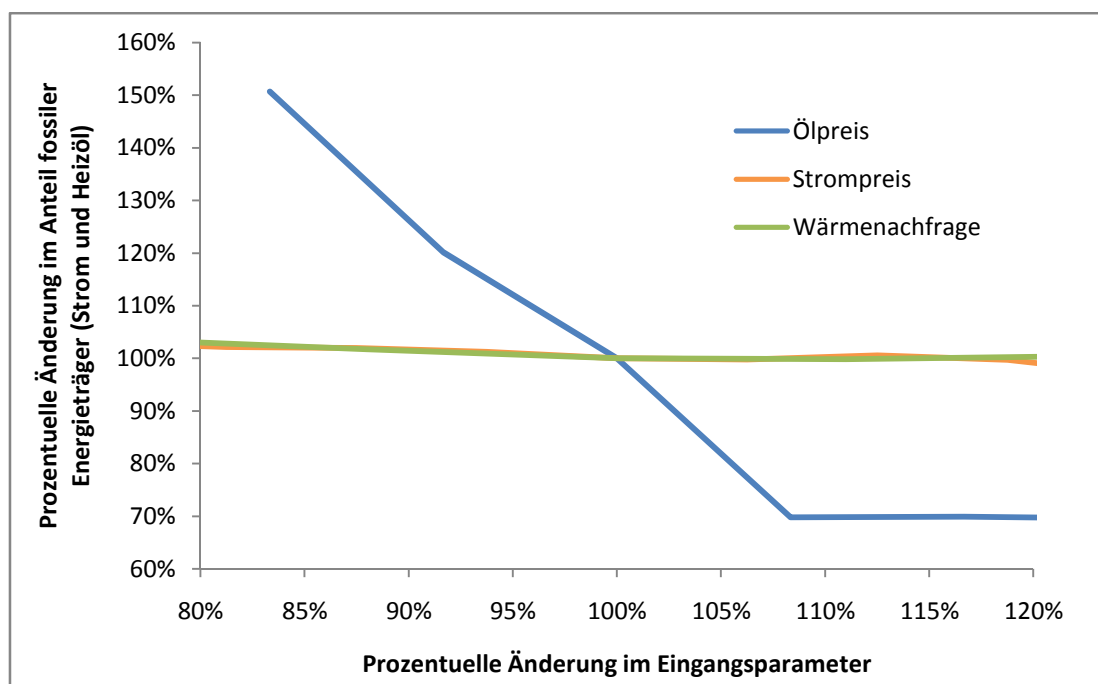
Abbildung 23 Sensitivität des Anteils von Heizöl und Netzstrom gegenüber Änderungen in den Inputparametern
