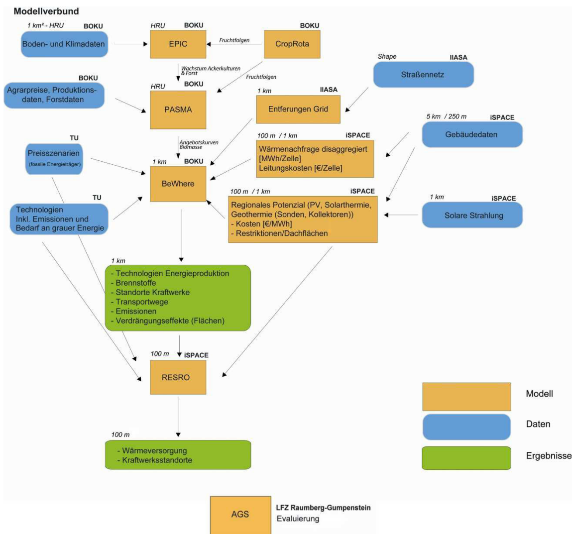
Abbildung 4 Gesamter Modellverbund
