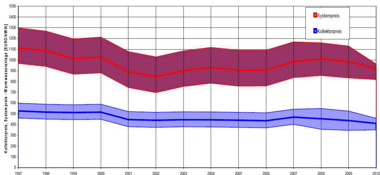
Abbildung 12 Repräsentative Bandbreiten der Systempreise und Kollektorpreise für Solarthermische Anlagen zur Warmwasserbereitung (Preise inflationsbereinigt mit der Basis 2010 und exkl. USt.) Quelle: AEE INTEC in Biermayr et al. (2011)
