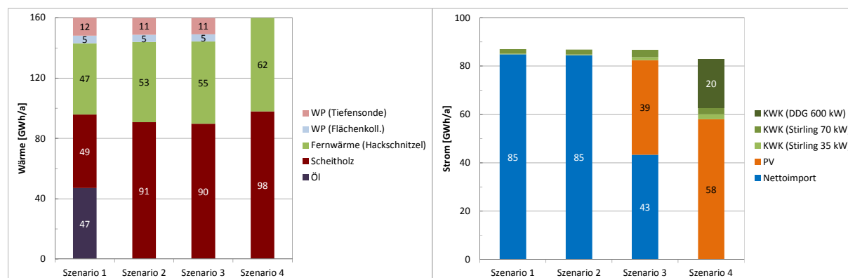
Abbildung 25 Wärmeezeugung auf Nutzenenergieebene (links) & Deckung des Strombedarfs (rechts)
