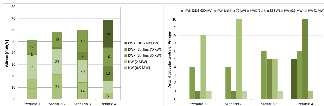
Abbildung 26 Wärme-Output (links) und Anzahl gebauter zentraler Bioenergieanlagen 13 (rechts) Kommentare: KWK-Angaben in elektrischer Leistung kW el , Heizwerk (HW)-Angaben in thermischer Leistung MW th . Die aufgeführten KWKs haben übrigens durch ihre sehr hohen Vollaststunden höhere Wärmeerzeugungskapazitäten als das HW mit 0,5 MW Leistung. Im linken Diagramm zum Wärme-Output sind bei den Kategorien HW auch bereits in der Region vorhandene Heizwerke integriert.
