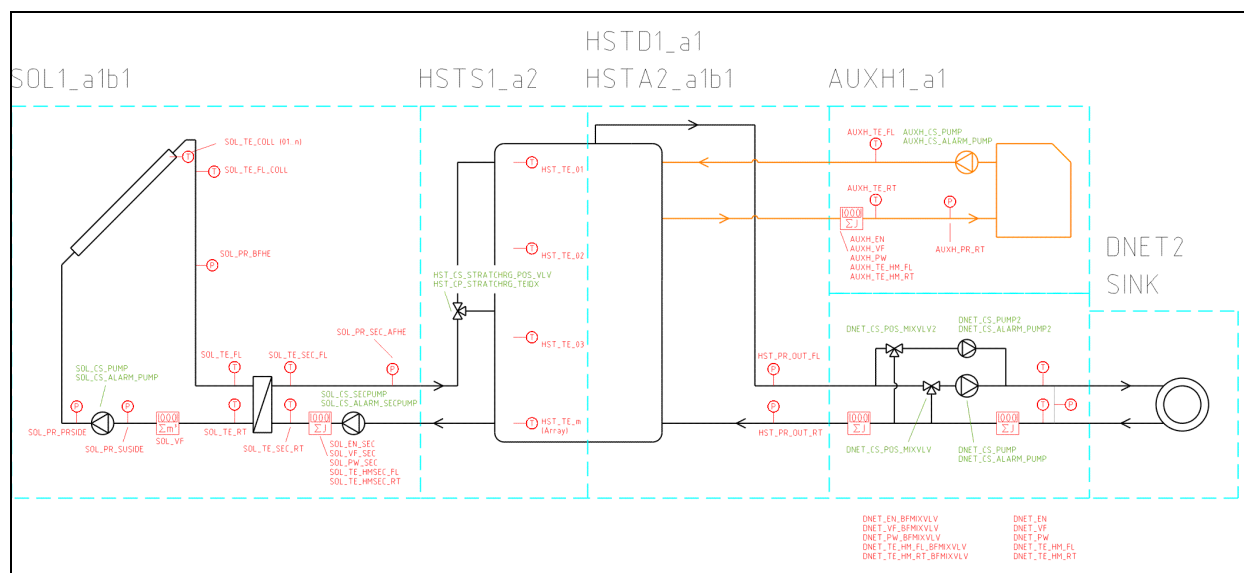
Abbildung 8 Pilotanlage „Krottendorfer Straße“, abgebildet an Hand der Ergebnissen aus AP 1, AP 2 und AP 4
