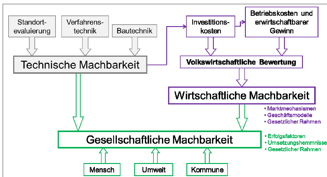
Abbildung 14: Fragestellungen der vertieften Machbarkeitsuntersuchung des Großwärmespeichers und Andeutung der Abhängigkeiten.
