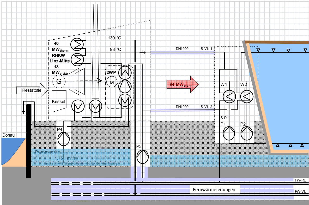
Abbildung 9: Reststoffheizkraftwerk mit angekoppelten Wärmepumpen und angeschlossenem Speicher.
