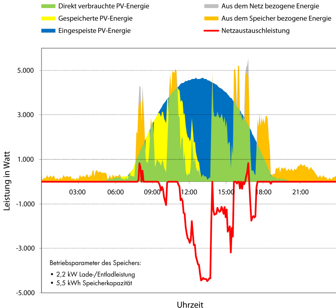
Abbildung 2: Reales Erzeugungs- und Verbrauchsprofil eines Haushalts mit 5,6kW PV-Anlage und 5,5kWh Speicher Daten SMA 2012 Quelle: /8/.
