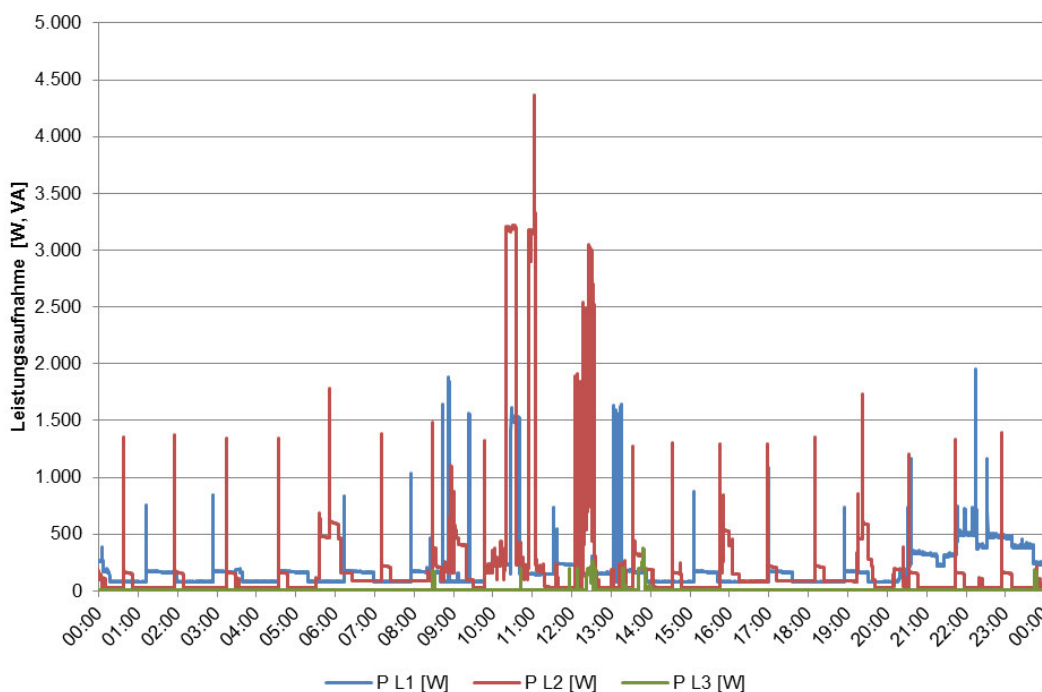
Abbildung 6: Messung der Phasenleistungsaufnahmen eines Haushaltes an einem Sommer-Sonntag; Messung im Rahmen von „ADRES-Concept“ Quelle:/11/.
