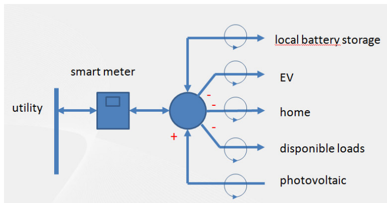
Abbildung 9: Micro Grid Zelle mit energy pools EP
