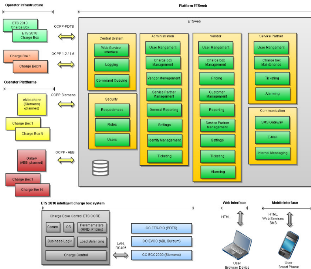
Abbildung 12: Software Architektur des ETSweb (www.enio.at)
