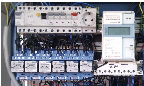
Abbildung 8: Testaufbau der Phasenauswahl-Schaltung mit einem HAGER Smart Meter
