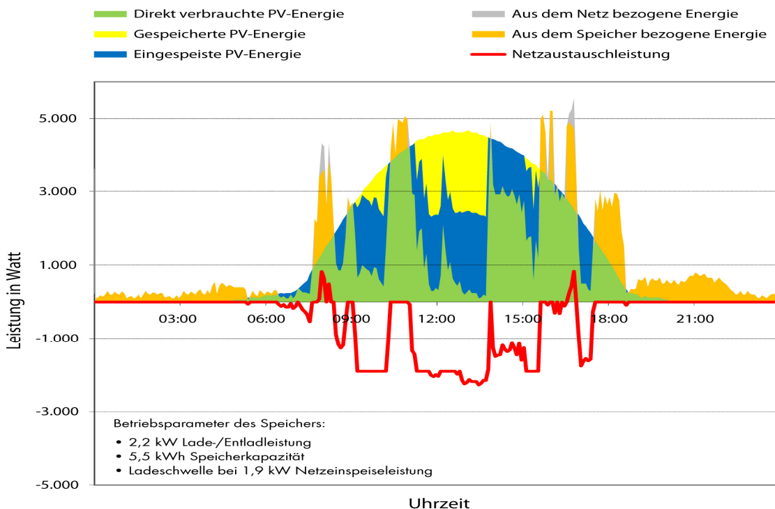
Abbildung 3: Lastausgleich durch gesteuerte Speicherung und Einspeisung. Erzeugungs- und Verbrauchsprofil eines Haushalts mit 5,6kW PV-Anlage, Daten SMA 2012 Quelle: /8/.
