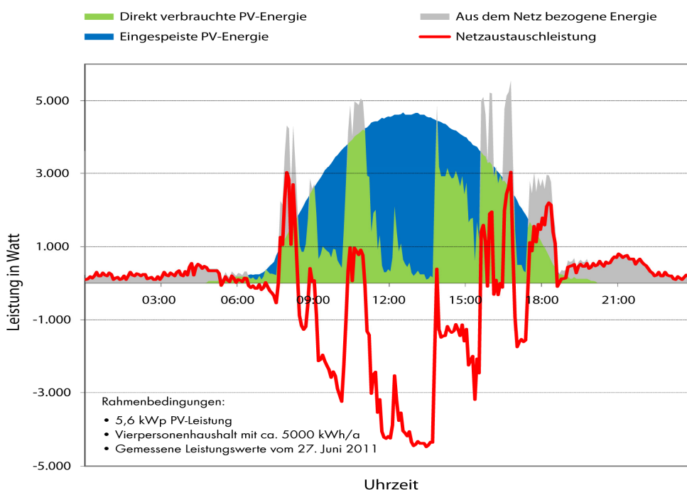
Abbildung 1: Vergleich der PV-Erzeugung (Blau) des Haushaltsverbrauchs Eigenverbrauch PV (Grün) + Netzbezug (Grau), sowie das ins Netz eingespeiste Energie-Netzaustauschleistung (Rot). Daten SMA 2012 /Quelle: /8/
