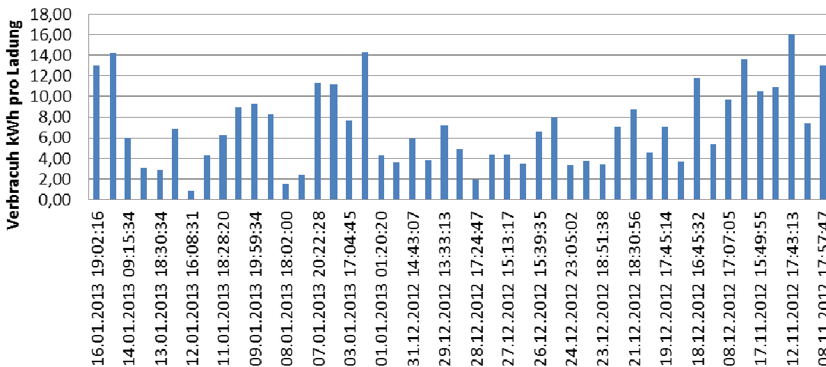
Abbildung 5: Energieverbrauch pro Ladevorgang. Auswertung aus 154 Ladevorgängen von 10 unterschiedlichen E-Fahrzeugen (Daten: PDT S GmbH 2012)
