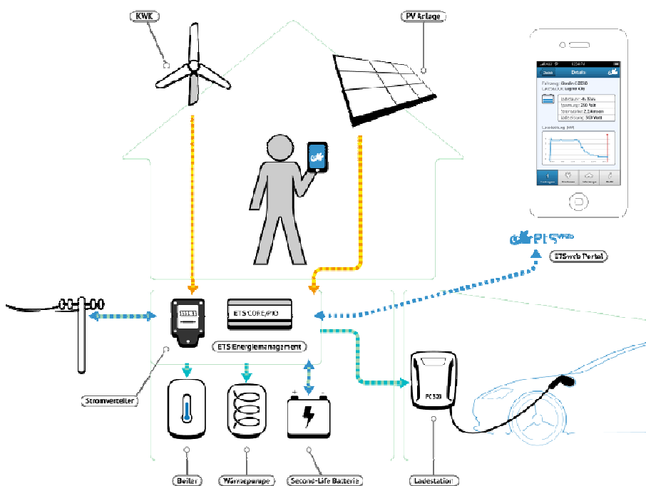
Abbildung 4: Energiemanagement durch ETS-CORE und Kommunikation mit PV-Anlage, Speichersystem und Fahrzeug. Installation im Stromverteilerkasten.
