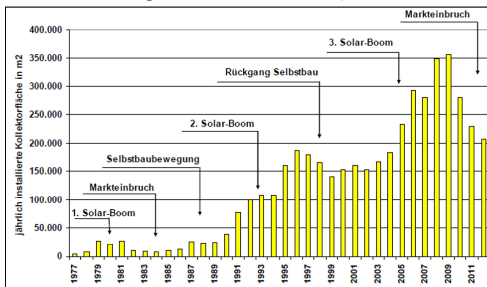
Abbildung 42: Solarwärmemarkt Österreich, 1977-2011
