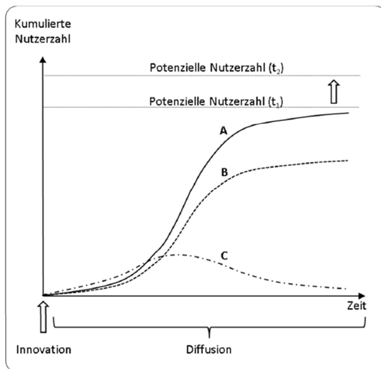
Abbildung 26: Stilisierte Diffusionsverläufe
