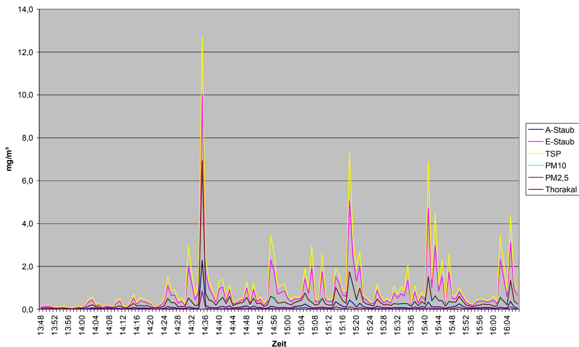
Abbildung 8 Staubentwicklung Situation A: A-Staub...alveolengängiger Staub, E-Staub...eintatembare Staub, TSP...Gesamtstaub in der Luft, PM10... Partikel kleiner 10 \mu\text{m} , PM2,5...Partikel kleiner 2,5 \mu\text{m} , Thorakal...Fraktion, die in und oberhalb der Bronchien deponiert wird
