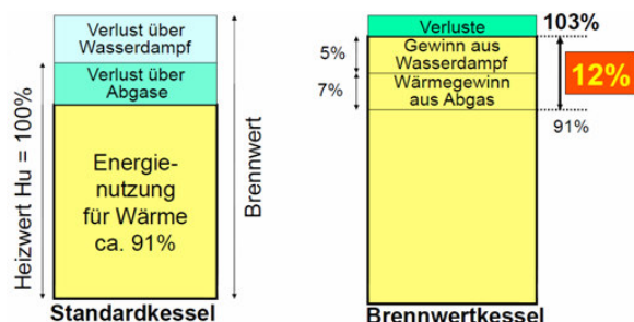
Abbildung 16: Energiegewinn durch Brennwerttechnologie 14
