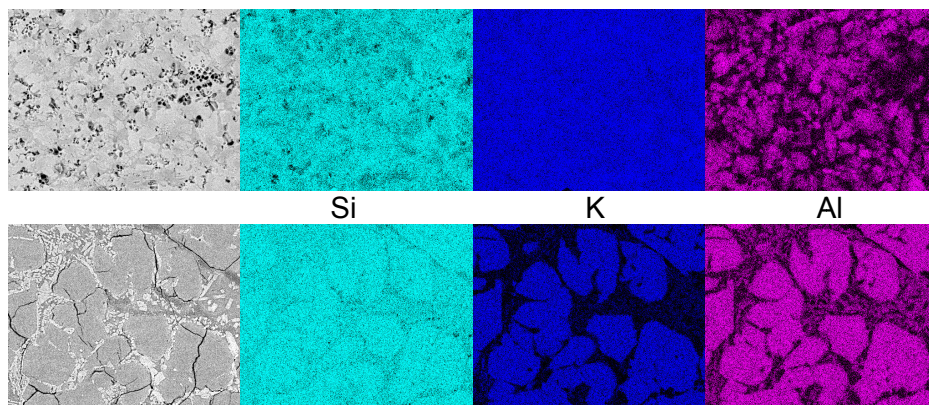
Abbildung 6: SEM/EDX-Analyse von Schlackeproben der Maisspindel-Testläufe
