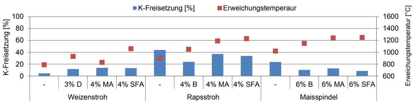
Abbildung 2: Zusammenfassung der Ergebnisse der Laborreaktortestläufe bzgl. K-Freisetzung und Erweichungstemperatur
