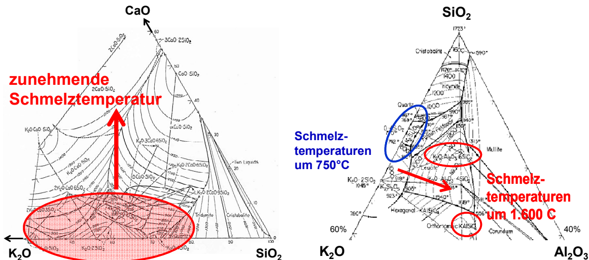
Abbildung 4: Ternäre Phasendiagramme CaO-K 2 O-SiO 2 und SiO 2 -K 2 O-Al 2 O 3
