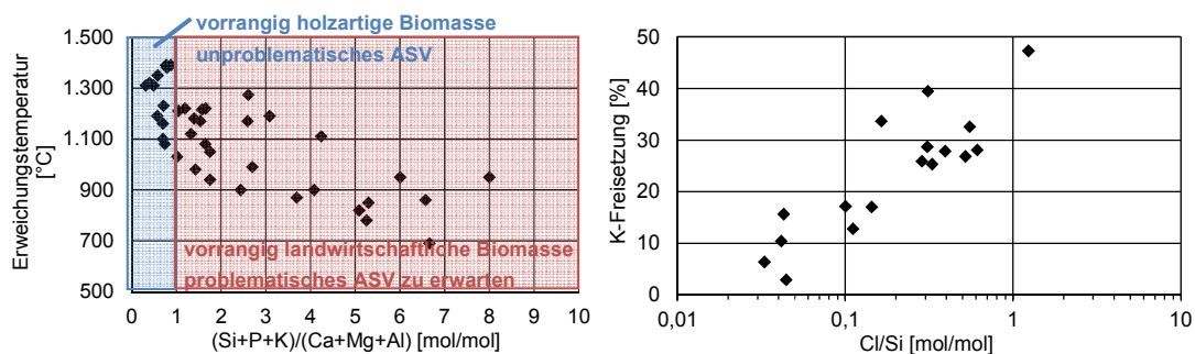
Abbildung 3: Erweichungstemperatur bzw. K-Freisetzungsfaktor vs. BSI
