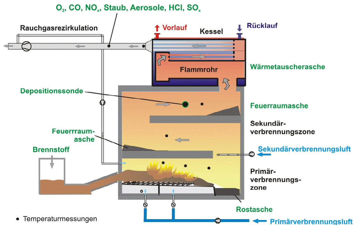
Abbildung 5: Schema der Feuerungsanlage mit Messstellen
