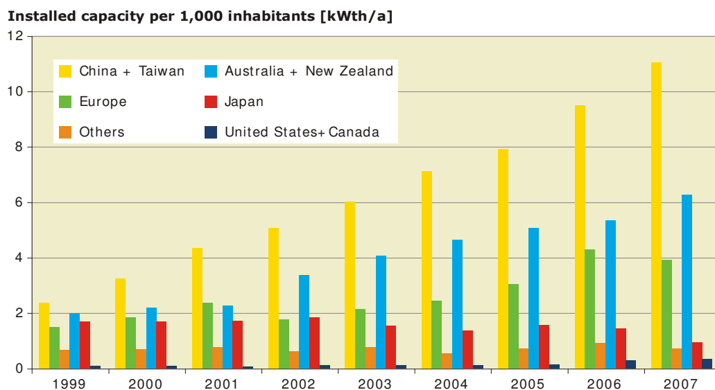
Abbildung 6: Jährlich neu installierte Leistung von Flach- und Vakuumröhrenkollektoren in kW th je Einwohner (Weiss, W. et.al.2009)
