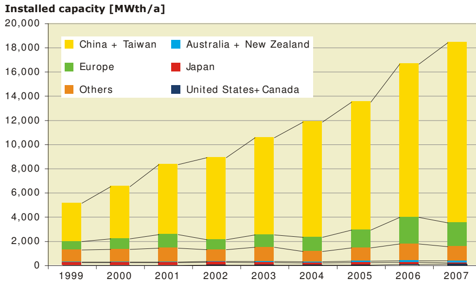
Abbildung 5: Jährlich neu installierte Kapazität von Flach- und Vakuumröhrenkollektoren in kW th , unterteilt nach Wirtschaftsregionen (Weiss, W. et.al.2009)
