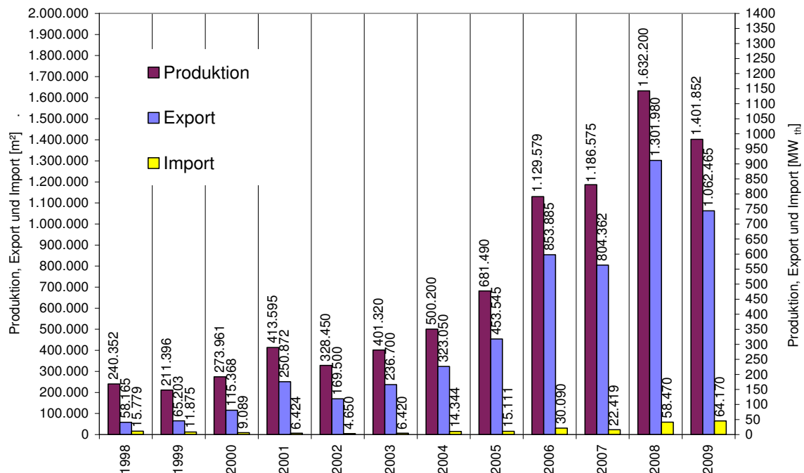
Abbildung 9: Export und Import von Kollektoren (Biermayr et.al.: BMVIT 2010)
