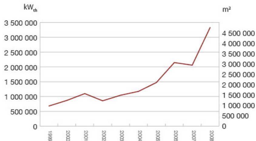
Abbildung 4: Marktentwicklung der Solarthermie in der Europäischen Union (ESTIF, 2009)
