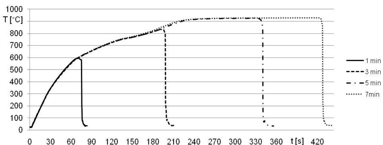
Abbildung 2: Bauteiltemperatur in Abhängigkeit der Ofenverweildauer, Ofentemperatur 920 °C
