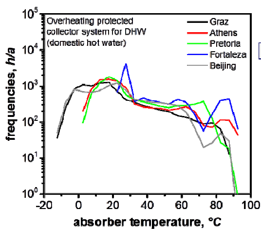
Abb. 4-4: Temperaturbelastungsprofile für den Absorber des AP-01-Kollektors (links) und zu erwartende Standort- abhängige Lebensdauern bei Einsatz der Werkstoffe PP-B1 und PP-B2 (rechts).
