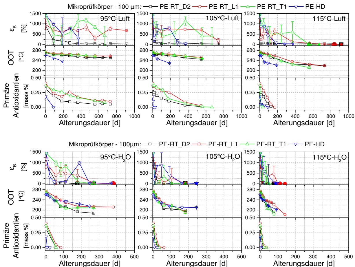
Abb. 5-1: Verläufe von Bruchdehnung \epsilon_B , Oxidationsonsettemperatur OOT und Konzentration primärer Antioxidantien für Mikroprüfkörper der Polyethylentypen PE-RT_D2, PE-RT_T1, PE-RT_L1 und PE-HD nach Alterung an Heißluft (oben) und in deionisiertem Wasser bei 95°C, 105°C und 115°C (unten) (Materialversprödung gekennzeichnet durch große, ausgefüllte Symbole).
