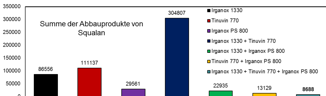
Abb. 5-2: Ranking von Stabilisatorsystemen bezüglich der thermooxidativen Beständigkeit einer PP-Modellsubstanz bei Heißluftlagerung.
