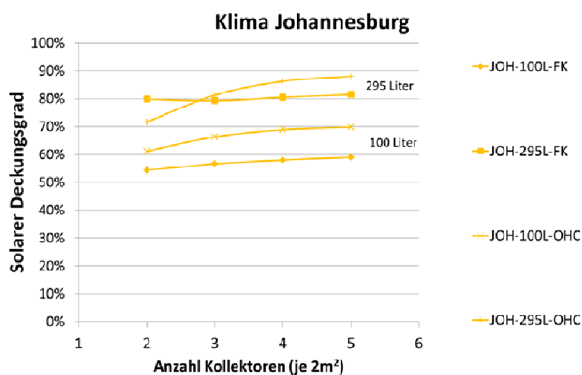
Abb. 1-3: Jahressimulation der Warmwasserbereitung mit sehr gutem Flachkollektor (FK; \eta_0=0,8 , a_1=3,0 ; a_2=0,01 ) im Vergleich zum Kunststoffkollektor mit Überhitzungsschutz (OHC; \eta_0=0,77 , a_1=6,1 ; a_2=0,007 ).
