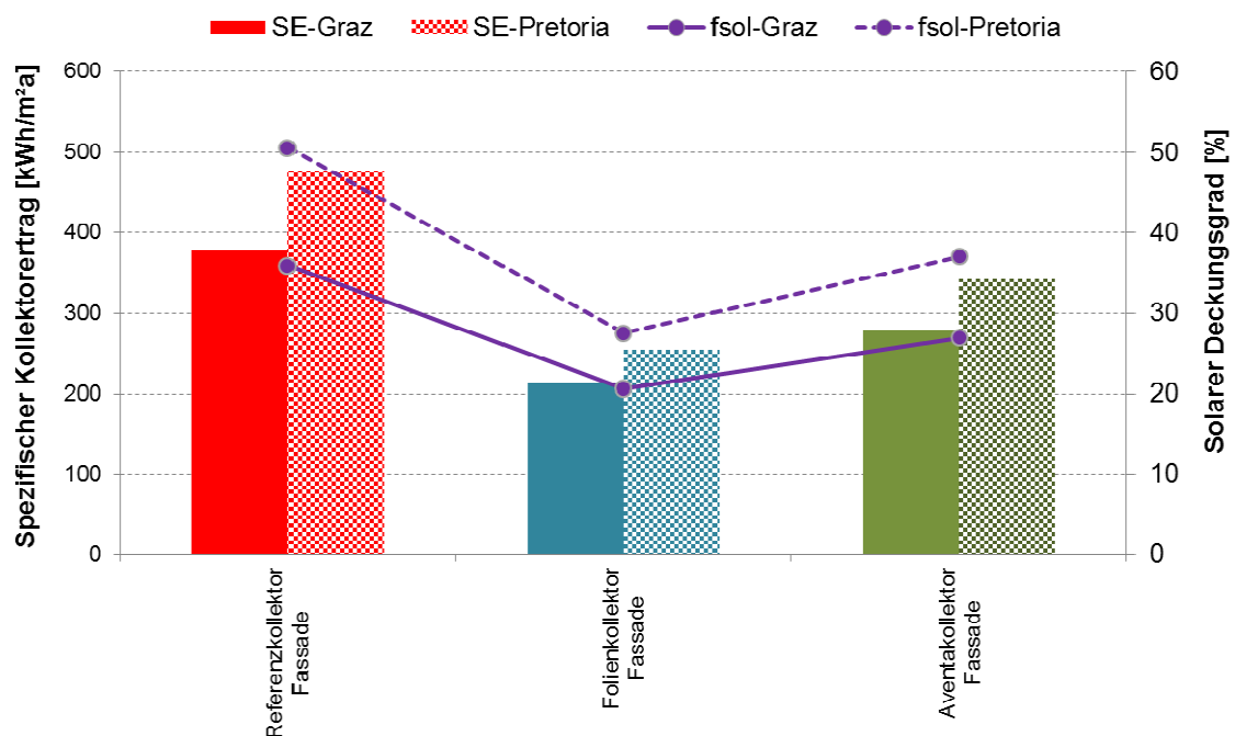
Abb. 3-2: Spezifischer Kollektorfeldertrag und solarer Deckungsgrad für fassadenintegrierte Warmwasserbereitungssysteme im Geschößwohnbau mit unterschiedlichen Kollektoren.
