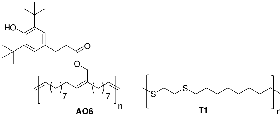
Abb. 4-1: Chemische Strukturen des synthetisierten makromolekularen phenolischen Anti-oxidants AO6 und des Oligomer-Thiosynergisten T1.
