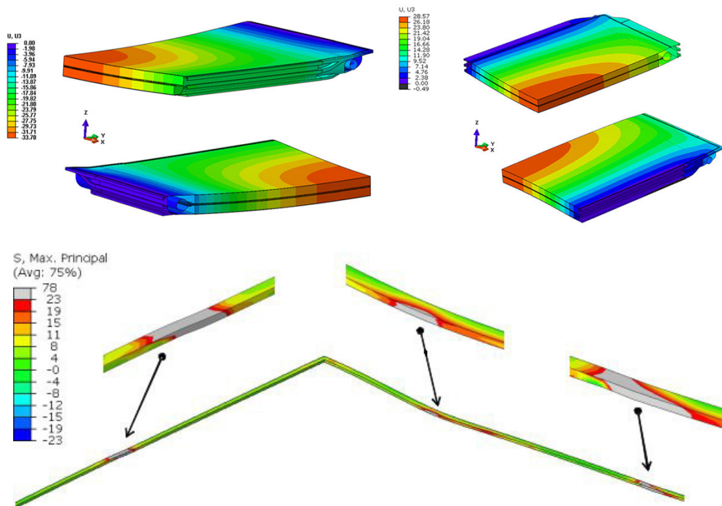
Abb. 2-2: Simulierte Spannungsverteilung bei Wind- und Schneelasten am Hybrid-Flachkollektor Sunlumo (oben) und in den Fügenähten zwischen transparenter Abdeckung und Rahmen (unten).
