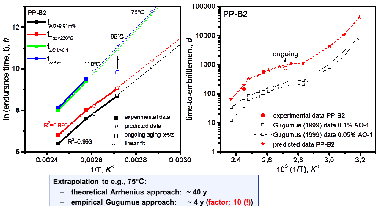
Abb. 4-3: Extrapolation der Alterungsindikatoren auf Einsatztemperaturen unter 100°C unter Verwendung des Arrhenius-Ansatzes (links) und des Gugumus-Ansatzes (rechts).
