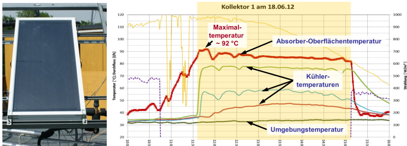
Abb. 1-1: Modell-Kollektor der Serie 1 am Prüfstand (links) und Verlauf der Kollektortemperaturen vor und nach dem Schalten des Ventils (rechts).
