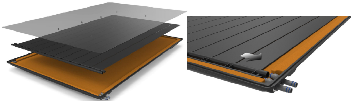
Abb. 2-1: Optimiertes Design für den Hybridflachkollektor Greiner mit ausgeschäumter Tiefziehwanne.
