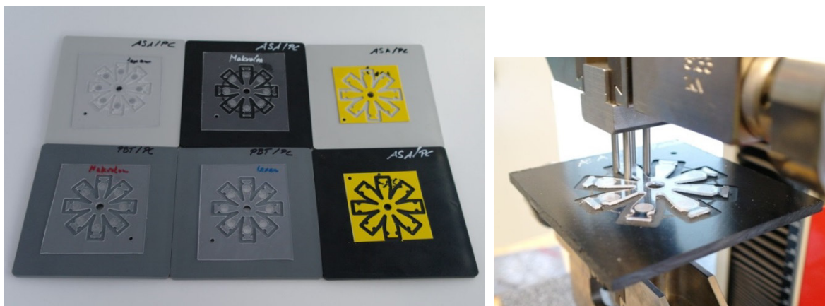
Abb. 2-3: Muster von lasergeschweißten Kunststoffpaarungen für das Kollektorgehäuse mit freigestellten Rosetten (links) für die reproduzierbare mechanische Charakterisierung (rechts).
