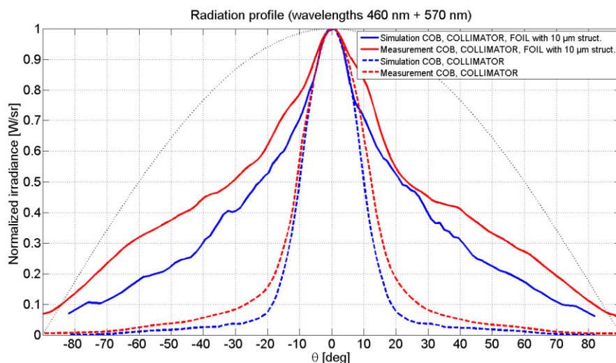
Abbildung 11: Simulierte und experimentell gemessene Abstrahlcharakteristika der Modul-Aufbauten (Kollimator mit und ohne Folienoptik).
