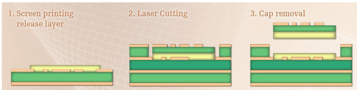
Abbildung 2: Grundsätzliches Verfahren zur Fertigung der Kavitäten im Leiterplattenmaterial.
