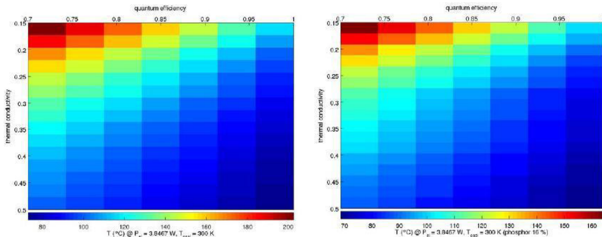
Abbildung 6: Oberflächentemperaturen auf der Farbkonversionsschicht während des Betriebs. Die linke Seite zeigt die Oberflächentemperatur für eine Farbkonversionsschicht eine Dicke von 400 µm und eine Phosphorkonzentration in der Silikonmatrix von 10 vol. % Durch Reduktion der Schichtdicke (200 µm) und Erhöhung der Phosphorkonzentration (16 vol. %) können die Oberflächentemperaturen deutlich reduziert werden (rechte Seite der Abbildung). Die Dicke und die Phosphorkonzentration der Farbkonversionsschicht wurden in letzterem Fall so gewählt, dass wiederum der gleiche Farbort des abgestrahlten weißen Lichts erreicht wird, wie im Fall der in der linken Seite dargestellt ist.
