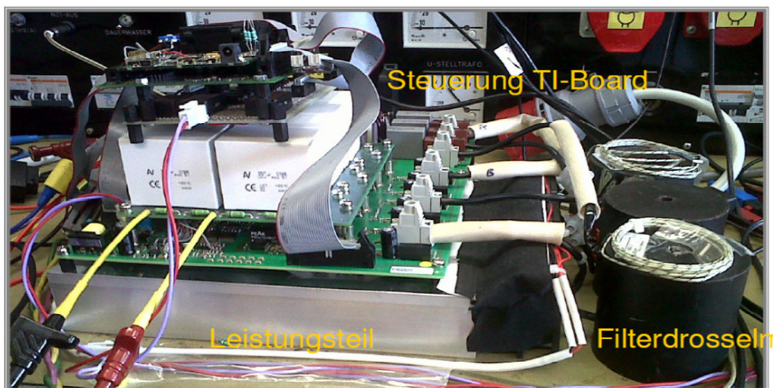
Abbildung 6: Prototyp 3-Level-NPC
