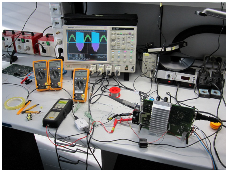
Abbildung 9 Schaltentlasteter 1~ Wechselrichterprototyp (3 kW Einspeiseleistung ins 230V-Netz)
