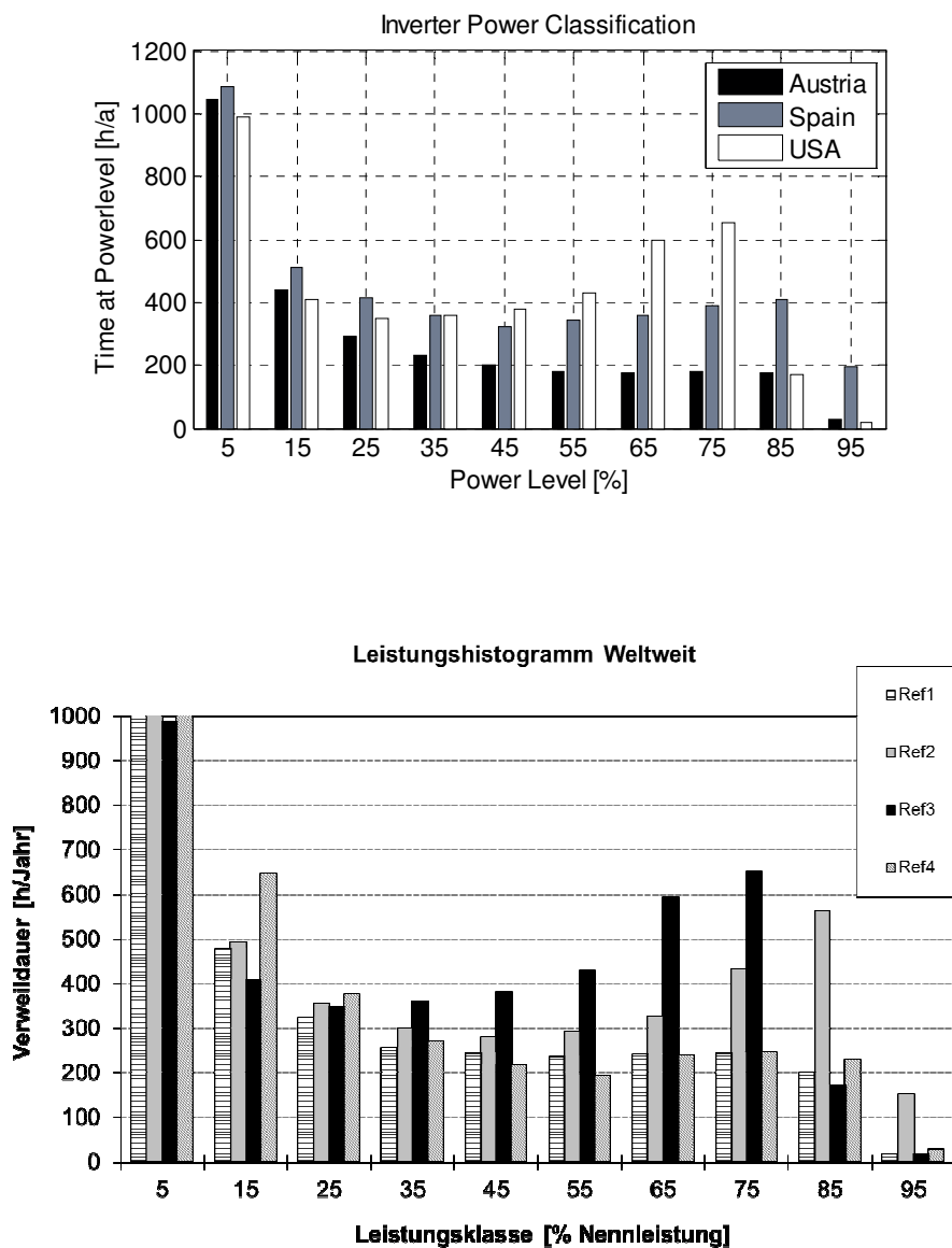
Abbildung 1: Leistungsklassen in verschiedenen Klimazonen
