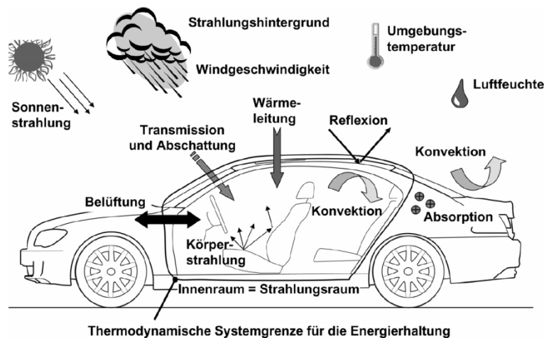
Abbildung 6: Übersicht über die physikalischen Zusammenhänge in einer Fahrgastzelle (Wagner, 2010)
