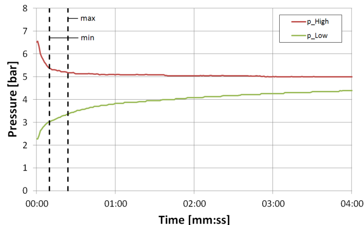
Abbildung 18: Verlauf von Hoch- und Niederdruck nach Abschaltung des Kompressors für OP 31 F bei 15 °C
