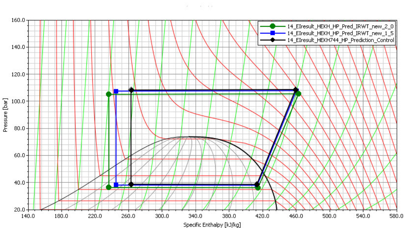
Abbildung 78: Auswirkung eines verbesserten Innenraumwärmetauschers (1,5- und 2,0-facher uA-Wert) auf den Prozess dargestellt im ph-Diagramm von R744
