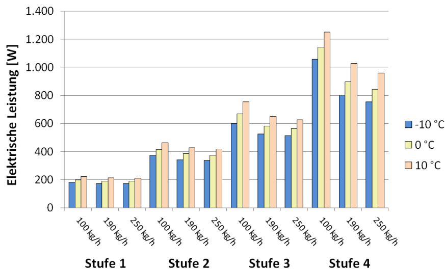
Abbildung 19: Elektrische Leistungsaufnahme des PTC-Heizelementes bei verschiedenen Betriebszuständen
