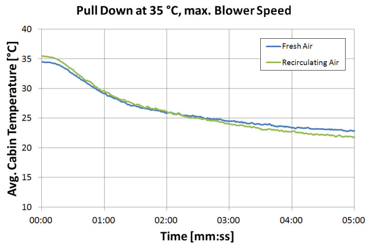
Abbildung 49: Mittlere Kabinentemperatur während des Abkühlversuches bei 35 °C
