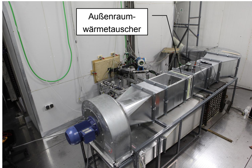
Abbildung 9: Luftkanal und aufgebaute Anlage in der äußeren Kammer
