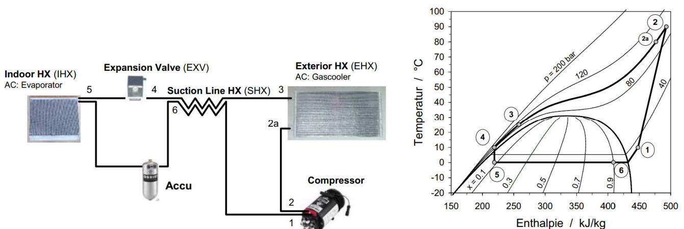
Abbildung 1: Prinzipschaltbild des typischen Aufbaus einer PKW-Klimaanlage mit \text{CO}_2 als Kältemittel (links) und schematischer Prozessverlauf im t/h-Diagramm (rechts) (Quelle: Lang et al., 2006)
