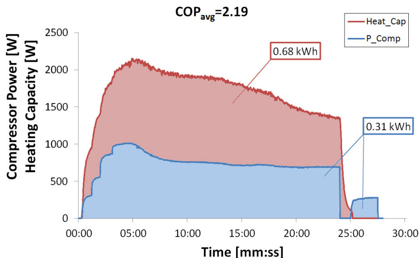
Abbildung 43: Energetische Betrachtung eines Vereisungs-Enteisungs-Zyklus
