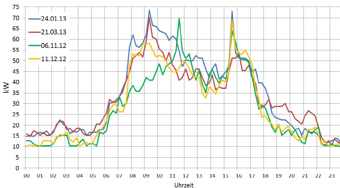
Abbildung 4: Darstellung des Lastverlaufs von Strom einer Schule an den Tagen mit der höchsten Leistungsspitze (Beobachtungszeitraum 1.9.2012 bis 31.8.2013).
