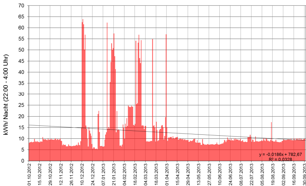
Abbildung 3: Darstellung des Stromverbrauchs in den Nachstunden (22:00 bis 4:00 Uhr) bei einem Objekt.
