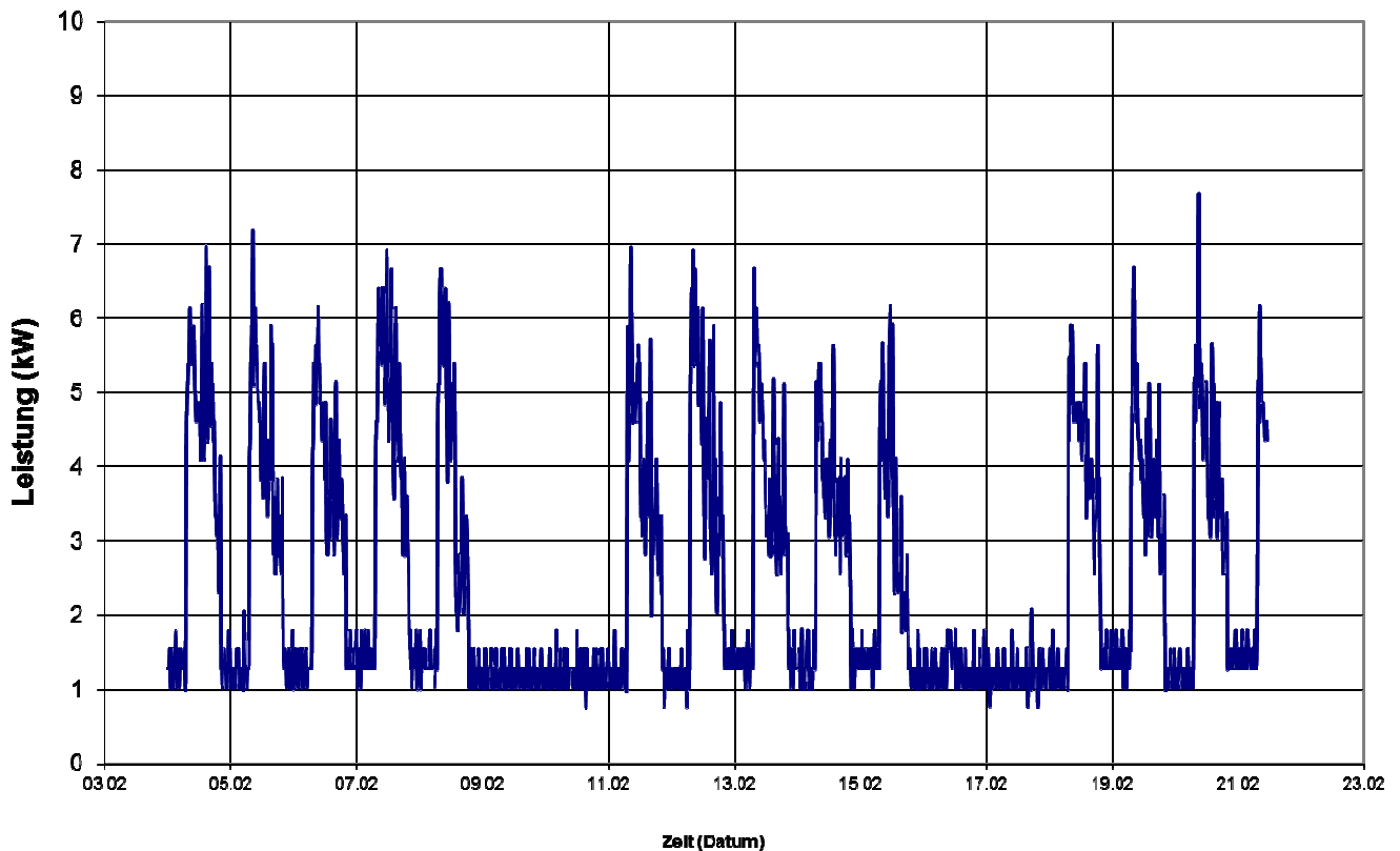
Abbildung 1: Lastverlauf eines Amtsgebäudes für den Zeitraum von 17 Tagen
