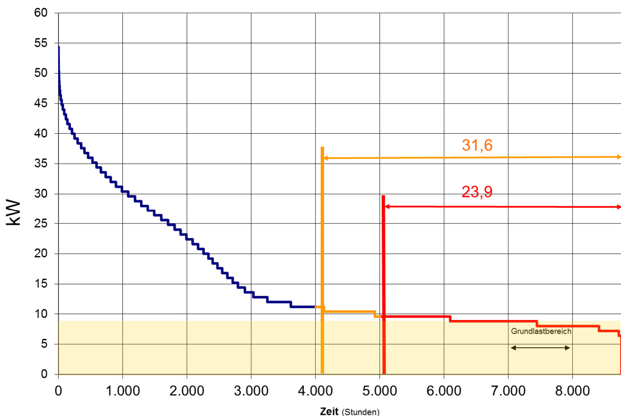
Abbildung 2: Geordneter Dauerlastgang eines Amtsgebäudes
