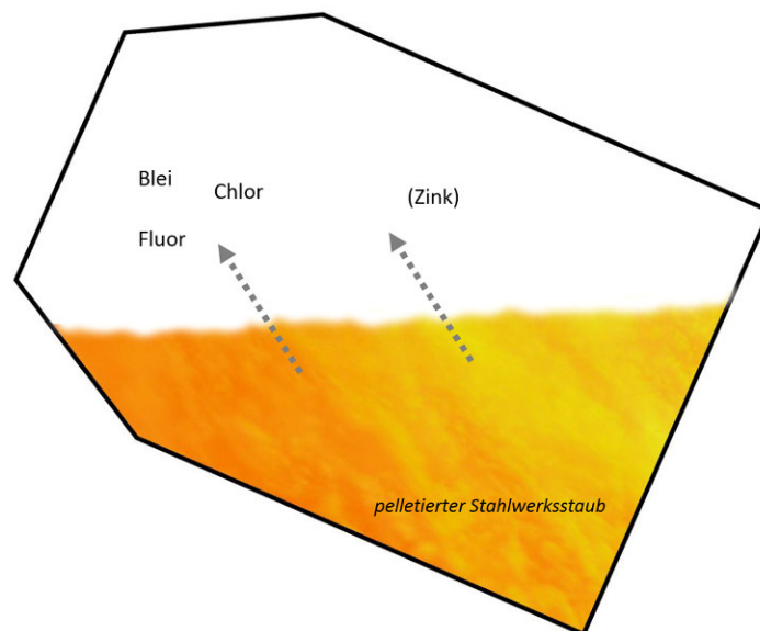
Abbildung 5: Schema der Klinkerstufe (Querschnitt eines TBRC Konvertergefäßes)
