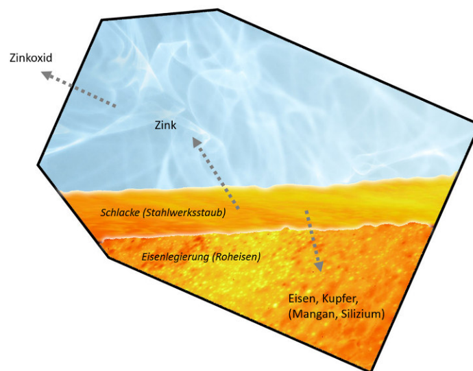
Abbildung 6: Schema der Reduktionsstufe (Querschnitt eines TBRC Konvertergefäßes)
