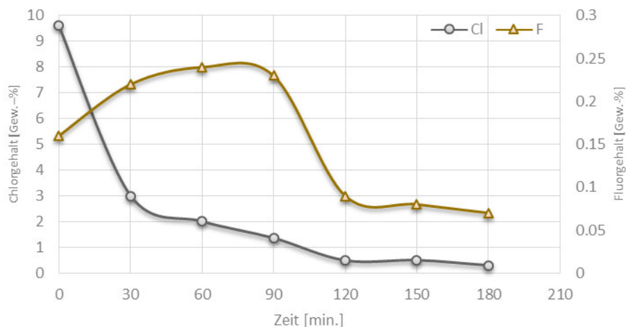
Abbildung 7: Verlauf der Halogenentfernung beim Klinkern
