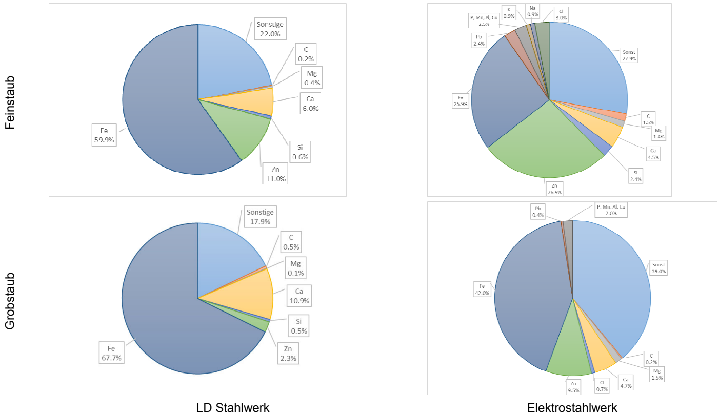
Abbildung 4: Durchschnittsanalyse verschiedener Stäube [7]
