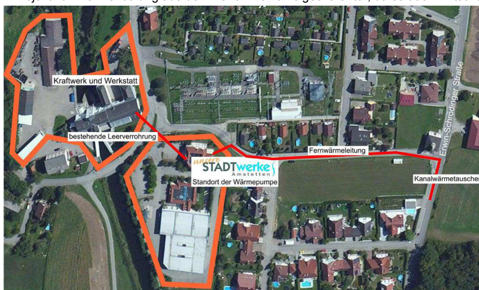
Abb.9:Amstetten, ein Projekt zur Wärmenutzung aus dem Kanal mit Vorzeigecharakter, da es auch wirtschaftlich rentabel ist
