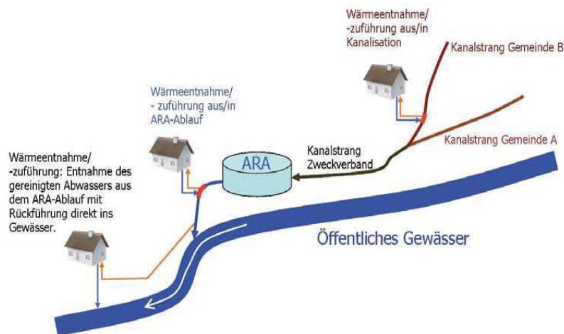
Abb. 1: Schematische Darstellung von Wärmeentnahmen und -einträgen
