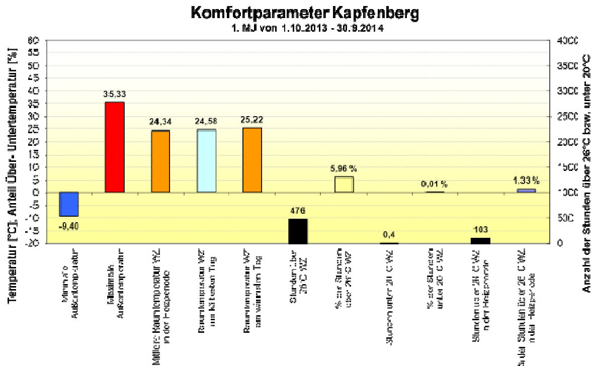
Abbildung 88 Überblick über die Komfortparameter in den Wohnzimmern der Johann-Böhmstraße 36 in Kapfenberg; gut ersichtlich ist die hohe Durchschnittstemperatur während der Heizperiode und die relativ geringe Stundenanzahl mit Temperaturen über 26°C im Sommer
