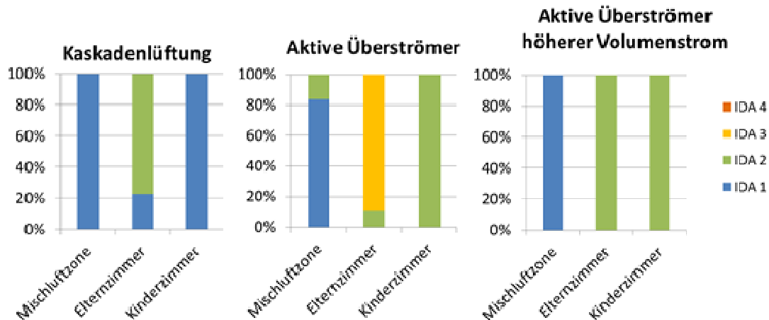
Abbildung 62 Simulationsergebnisse für die Luftqualität (CO 2 -Konzentration) nach Häufigkeit in den jeweiligen 4 IDA-Klassen nach [63] klassifiziert, bei Belegung der jeweiligen Räume. Links für ein „übliches“ Kaskadenlüftungskonzept, Mitte für das gemessene Konzept mit aktiven Überströmelementen und rechts mit aktiven Überströmelementen und höheren Volumenströmen.
