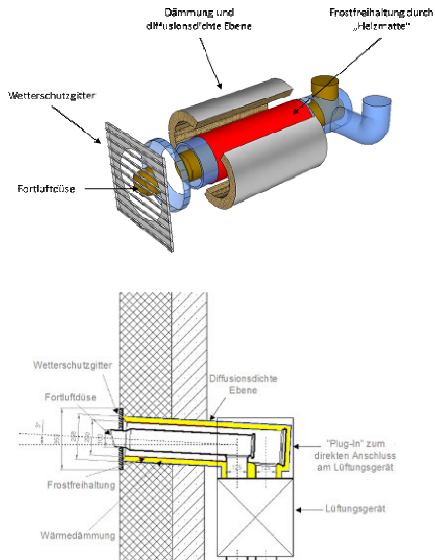
Abbildung 39 Skizzen des Koaxialrohres und der Frostschutz “Heizmatte” in SktechUp und in CAD als Vorlage für das Funktionsmuster.
