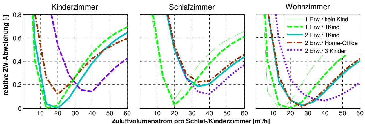
Abbildung 29 Relative Zielwertabweichung in Kinder-, Schlaf- und Wohnzimmer bei Variation der Zuluftmenge der Schlafräume für die beschriebene Referenzwohnung ohne Wohnzimmerzuluft für verschiedene Belegungsszenarien.
