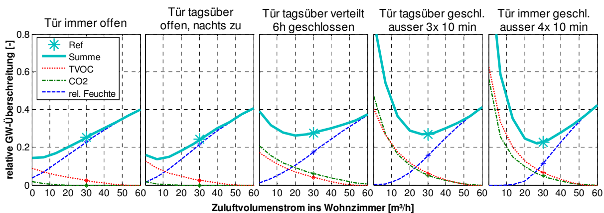
Abbildung 28 Raumluftqualität bei Variation des Zuluftvolumenstroms in ein vom Flur abgetrenntes Wohnzimmer für verschiedene Türöffnungsprofile.
