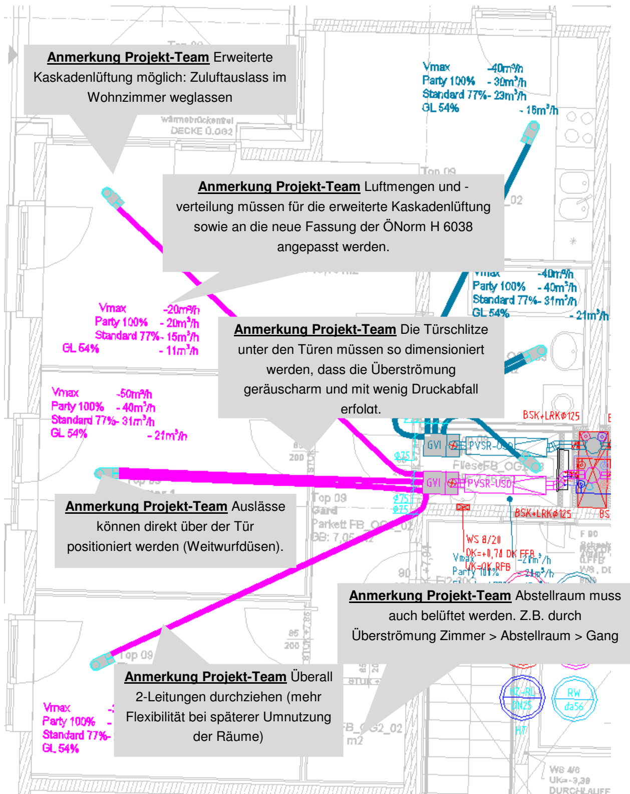
Abbildung 78 Detail aus dem Plan ACAD-3OG_HLS.dwg vom HLS Planung, Stand 10.04.2013
