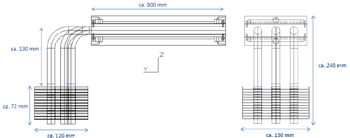
Abbildung 55 CAD Zeichnung vom Funktionsmuster der Heatpipe (Quelle: Fa. Dau).
