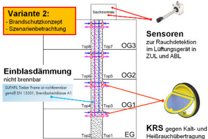
Abbildung 140 Brandschutzlösung - Variante 2
