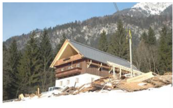
Abbildung 5: neuer Dachstuhl samt neuer Dachdeckung
