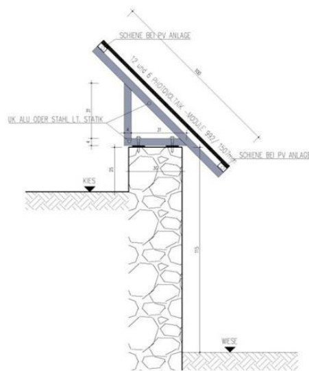
Abbildung 64: Schnitt durch Anlage 3
