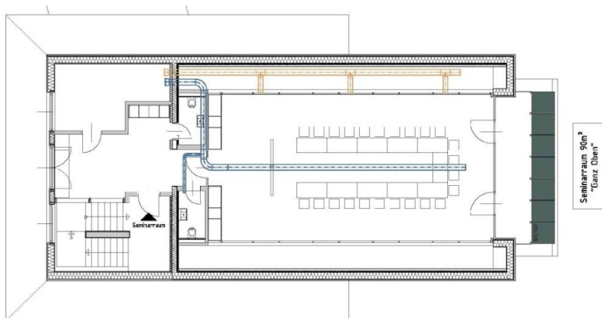
Abbildung 49: Lüftungsplan Dachgeschoß: Zuluftkanäle aus Zirbenholz (braun), Abluftkanäle aus Metall (blaugrau)
