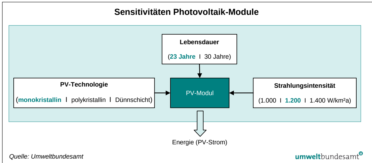
Abbildung 33: Varianten im Bereich Photovoltaik für das betrachtete Elektrofahrzeug (fett gedruckt: Standardtechnologie).
