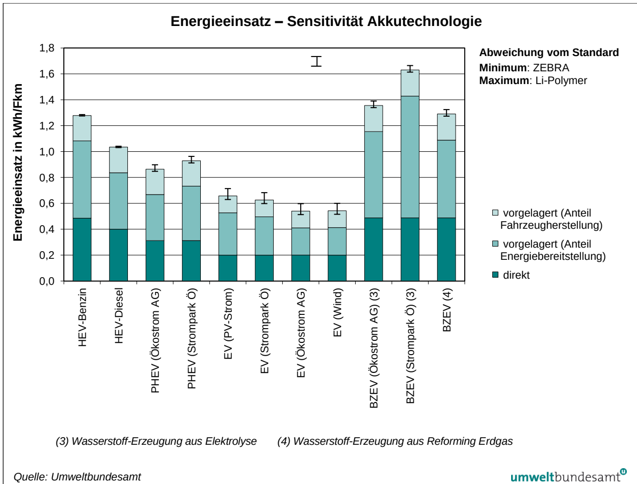
Abbildung 32: Gesamter Energieeinsatz für verschiedene Elektrofahrzeuge und Abweichung der verschiedenen Akku-Technologien (LiFePO 4 , Li-Polymer, ZEBRA) von der Standard-Technologie (Li-Ionen).
